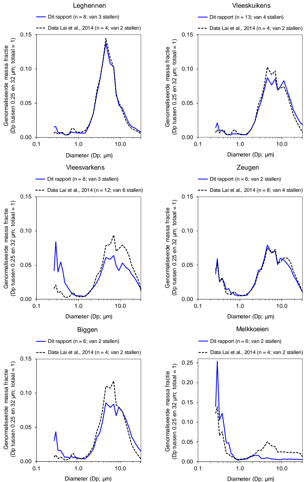
Figuur 3 Massafractie als functie van de deeltjesdiameter
