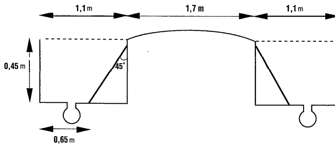
Figuur 2: Dwarsdoorsnede biggenopfoekafdeling met schuine putwanden
