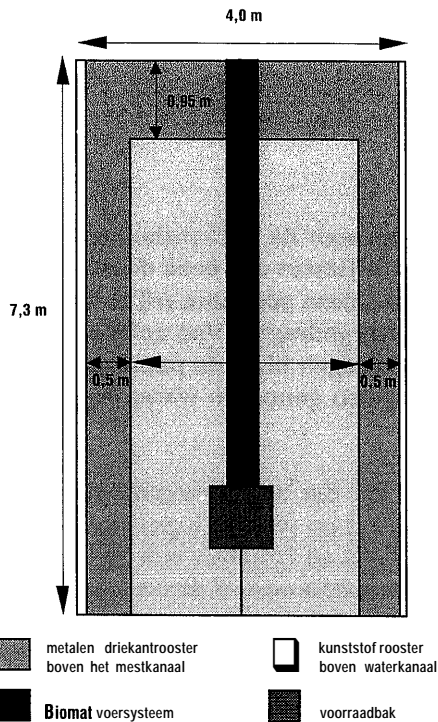
Figuur 1: Biggenopfoekafdeling met gescheiden water- en mestkanaal
