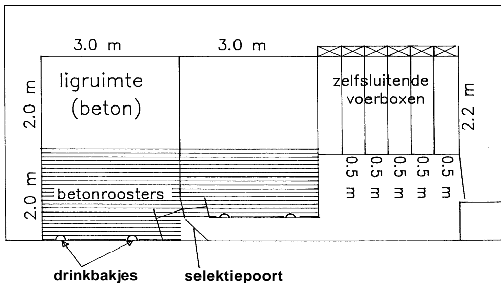
Figuur 1: Plattegrond van de experimentele loopstal-opstelling op het Proefstation voor de Varkenshouderij te Rosmalen
