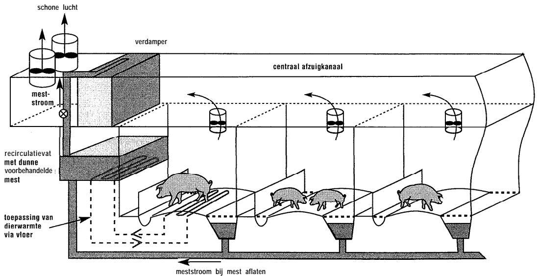
Figuur 1: Mogelijke uitvoering van een geïntegreerd luchtbehandelingssysteem
