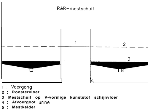
Figuur 1: Dwarsdoorsneden van de vijf onderzochte systemen
