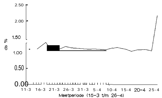
Figuur 3 Verloop droge-stofgehalte in het speelwater
