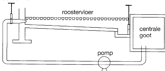
Figuur 1 Spoelsysteem wachtruimte
