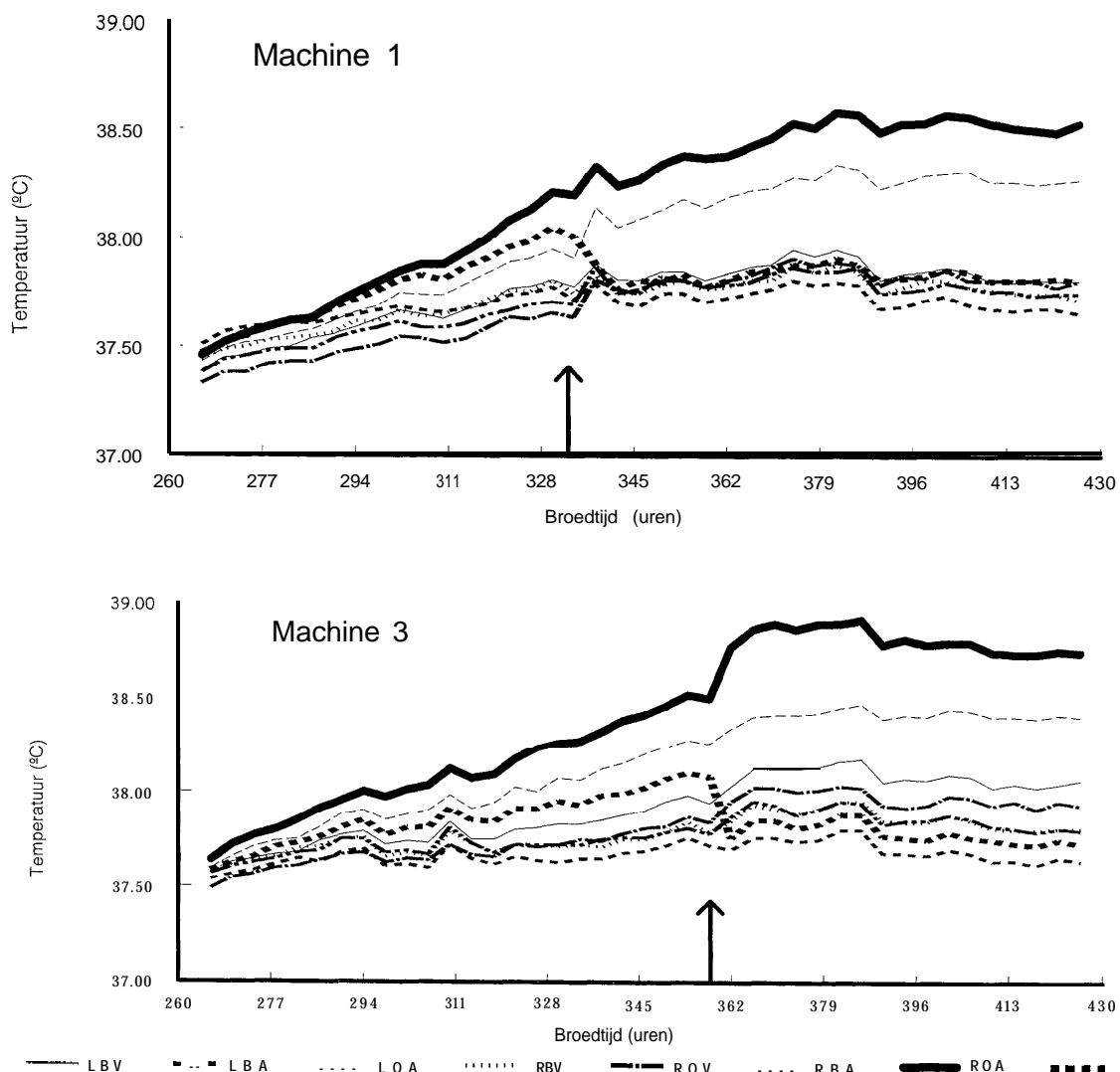
Figuur 2. Eischaltemperatuur ( ^{\circ}\text{C} ) in de verschillende compartimenten vanaf 11 dagen broeden tot aan het moment van overleg. In machine 1 werd na 336 uur gestopt met keren, in machine 3 na 360 uur. Indeling compartimenten: links (L) en rechts (R), boven (B) en onder (O), voor (V) en achter (A).
