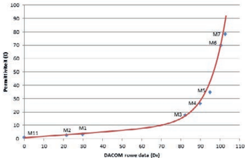
Figuur 2.7 Sensorkalibratie voor de Sensetion. Het verband tussen de ruwe meetwaarde ( D_R ) en de permittiviteit ( \epsilon ) voor verschillende kalibratie vloeistoffen (M1 – M7) en in lucht (M11), gemeten bij 25°C.
