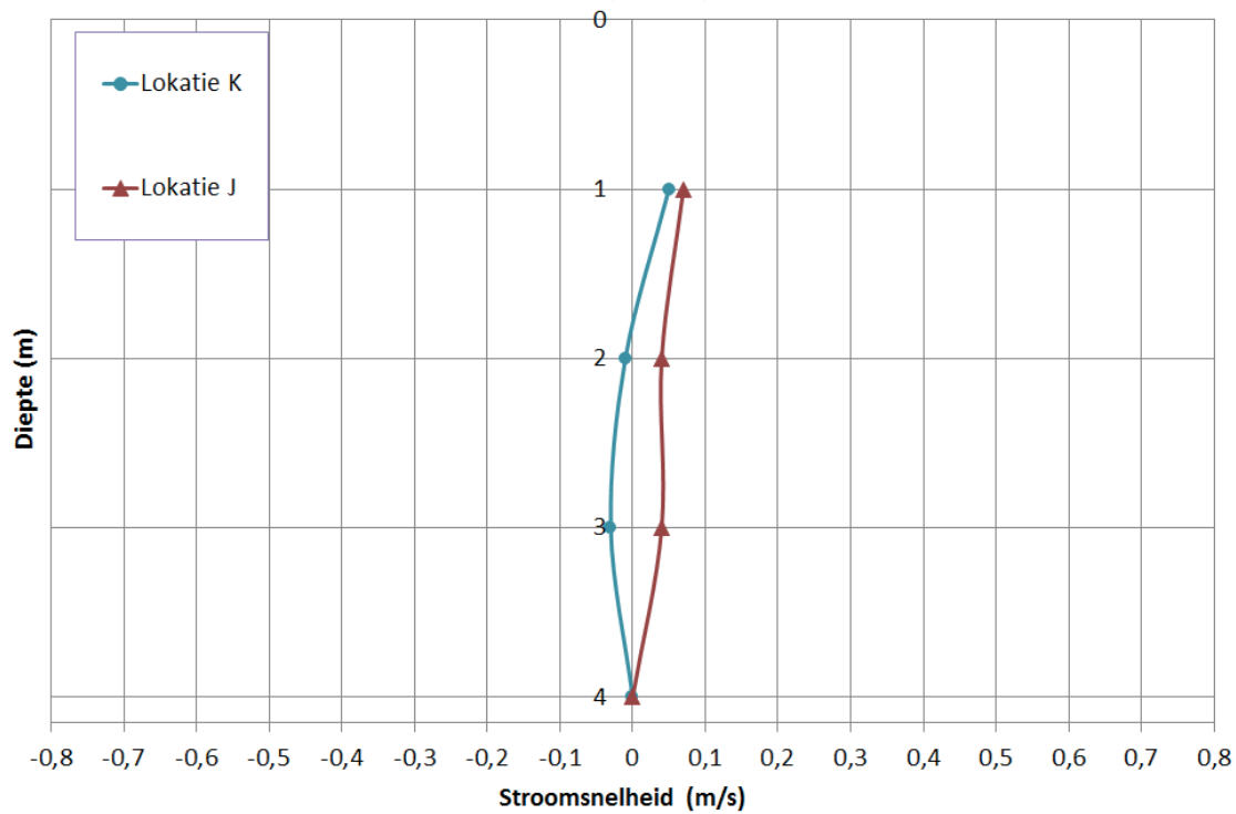
AFBEELDING 3.10 STROOMSNELHEDEN TUSSEN DE BELUCHTINGSPAKKETTEN (Z-RICHTING)
