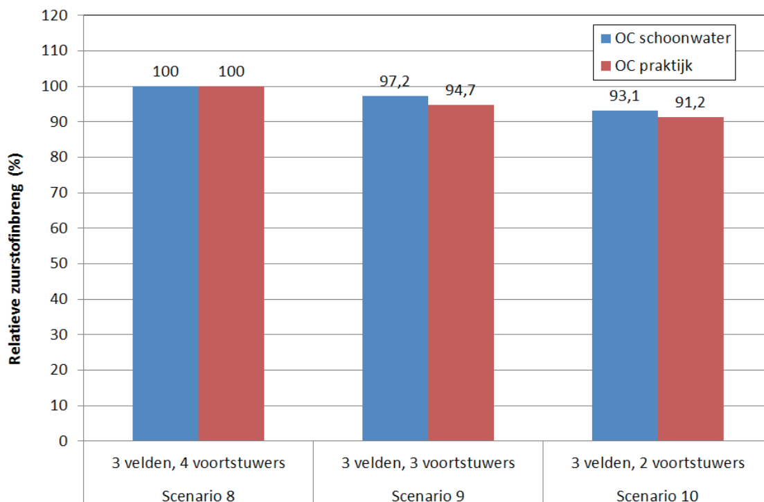
AFBEELDING 34 RELATIEVE ZUURSTOFINBRENG IN SCHOONWATER EN IN DE PRAKTIJK (75% BELUCHTING)
