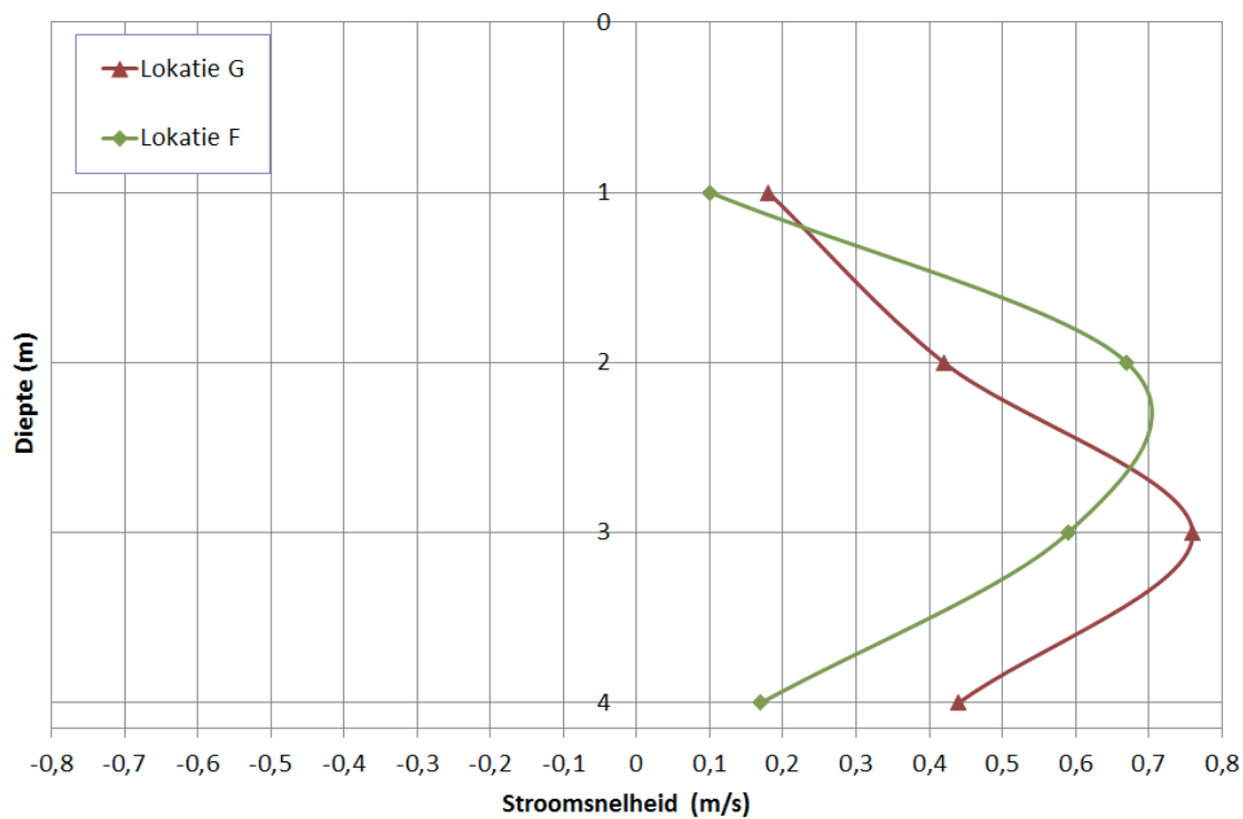
AFBEELDING 2.5 STROOMSNELHEDEN STROOMOPWAARTS VAN HET BELUCHTINGSPAKKET (X-RICHTING)
