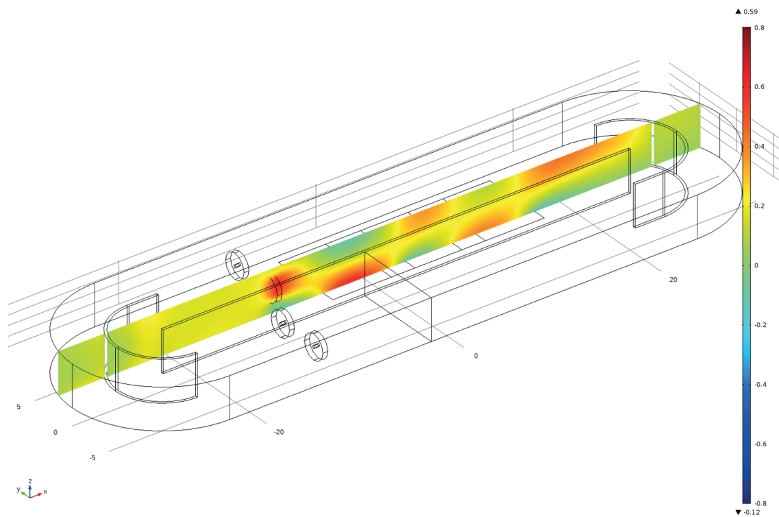
AFBEELDING 5.10 DOORSNEDE SNELHEID IN DE LENGTERICHTING (SCENARIO 12)
