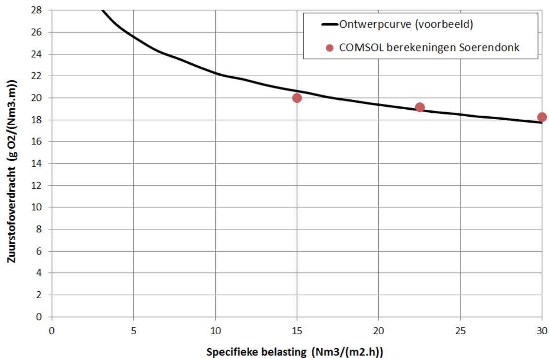
AFBEELDING 29 ZUURSTOFOVERDRACHT VERSUS PLAATBELASTING
