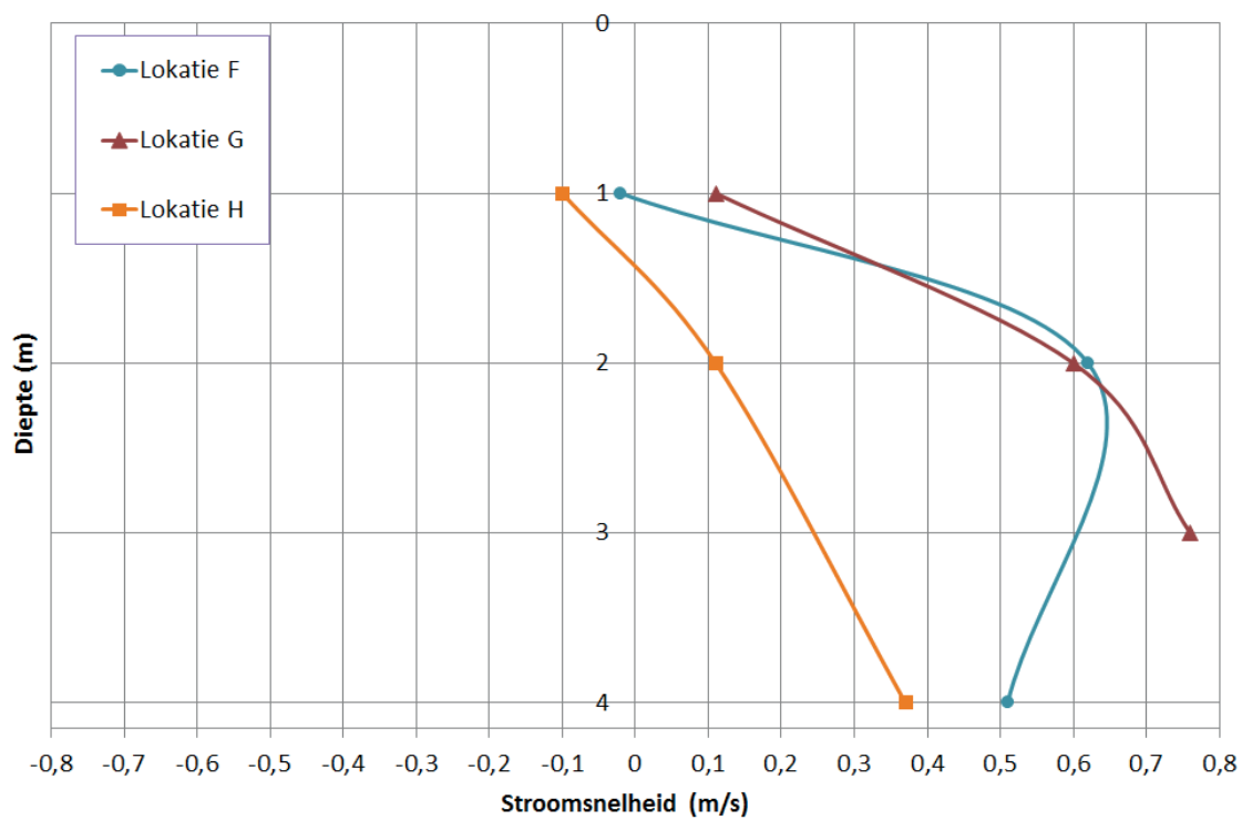
AFBEELDING 3.6 STROOMSNELHEDEN STROOMOPWAARTS VAN HET BELUCHTINGSPAKKET (Y-RICHTING)
