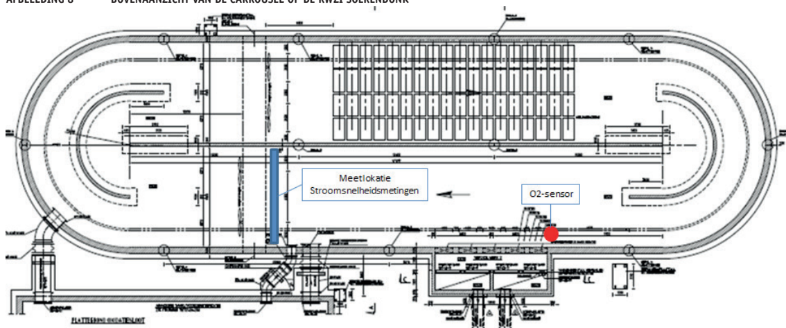
AFBEELDING 8 BOVENAANZICHT VAN DE CARROUSEL OP DE RWZI SOERENDONK
