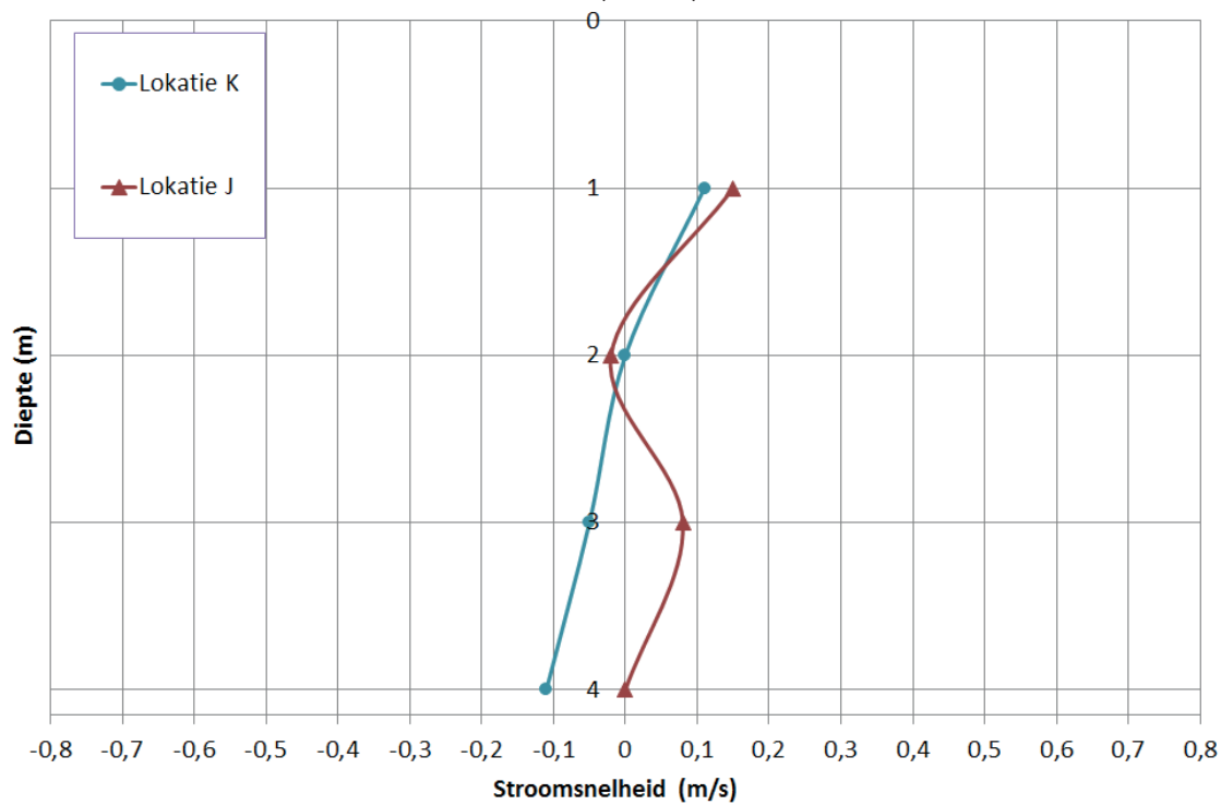
AFBEELDING 3.9 STROOMSNELHEDEN TUSSEN DE BELUCHTINGSPAKKETTEN (Y-RICHTING)
