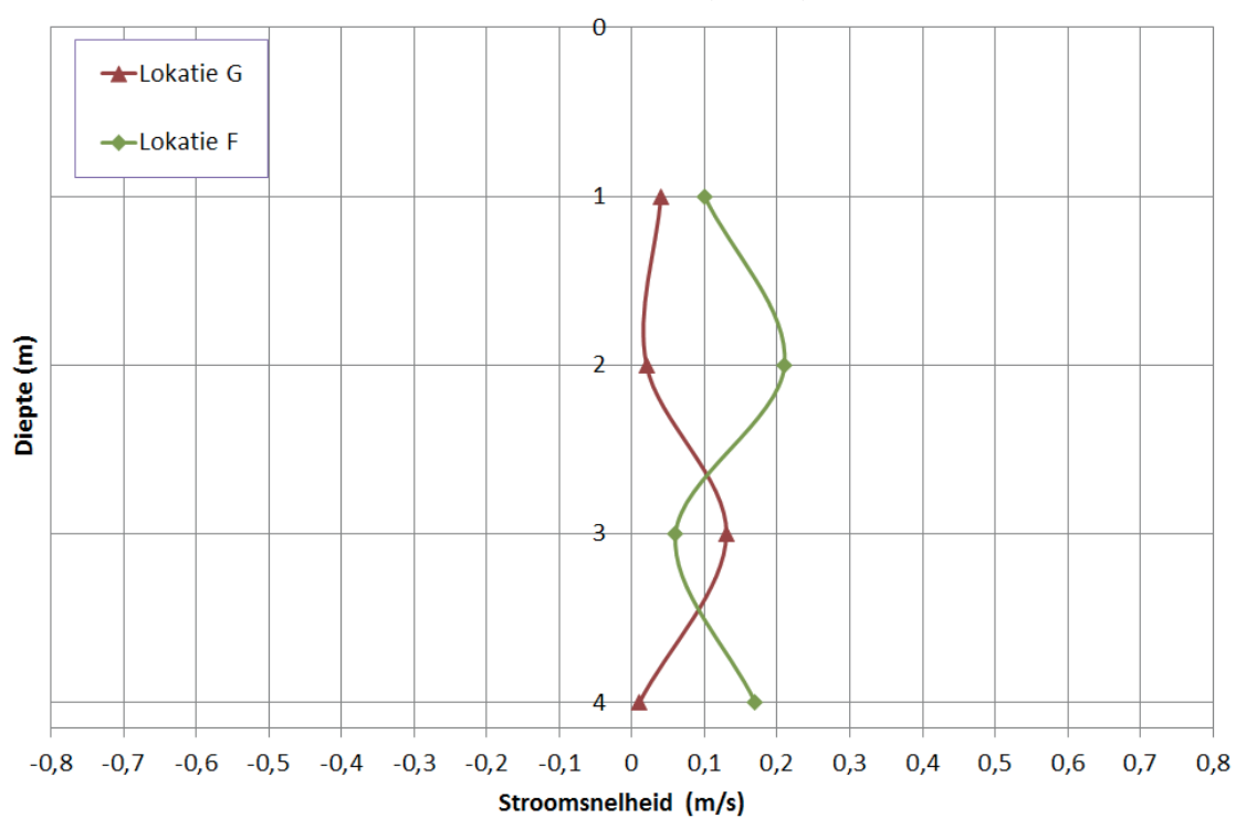
AFBEELDING 2.6 STROOMSNELHEDEN STROOMOPWAARTS VAN HET BELUCHTINGSPAKKET (Y-RICHTING)
