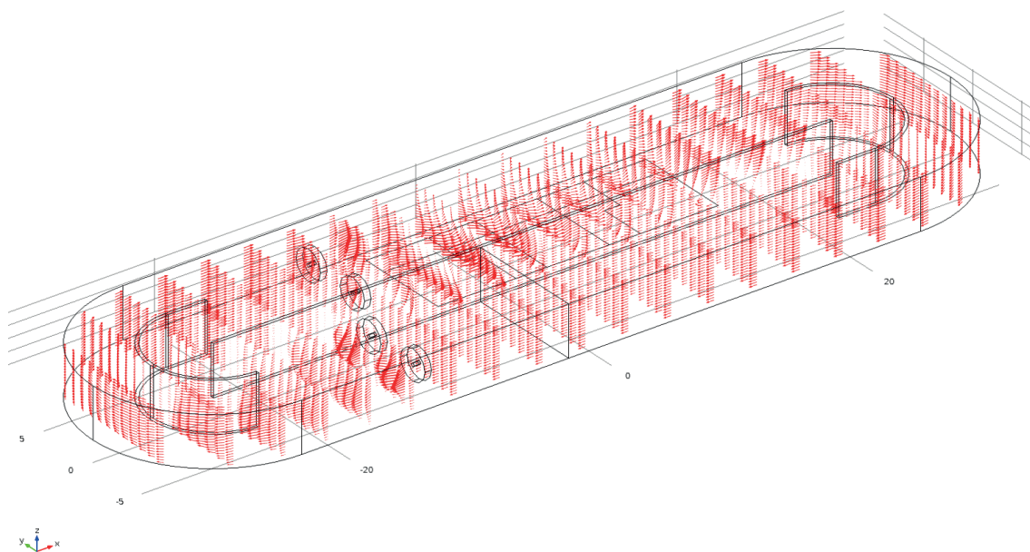
AFBEELDING 5.4 SNELHEIDSVECTORVELD SCENARIO 11
