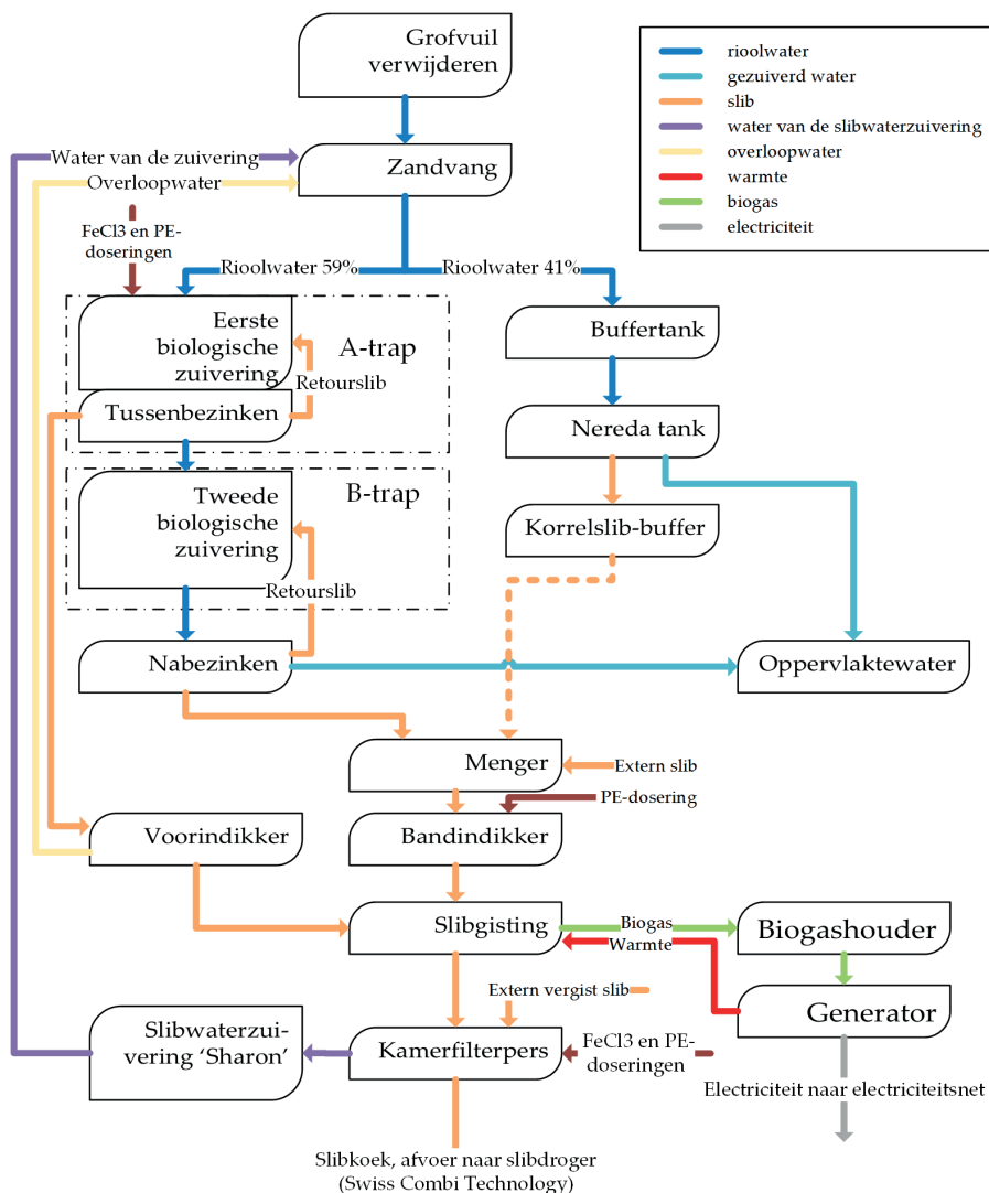
SCHEMATISCHE WEERGAVE VAN DE WATER- EN SLIBLIJN VAN RWZI GARMERWOLDE
