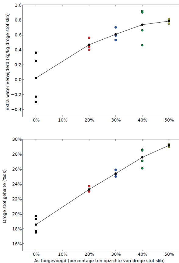
FIGUUR 65 ONTWATERING MET AS MET 65 G/KG DS FeCl_3
