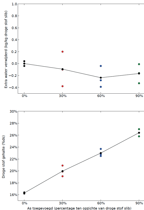
FIGUUR 64 ONTWATERING MET SLIBAS ZONDER FeCl_3
