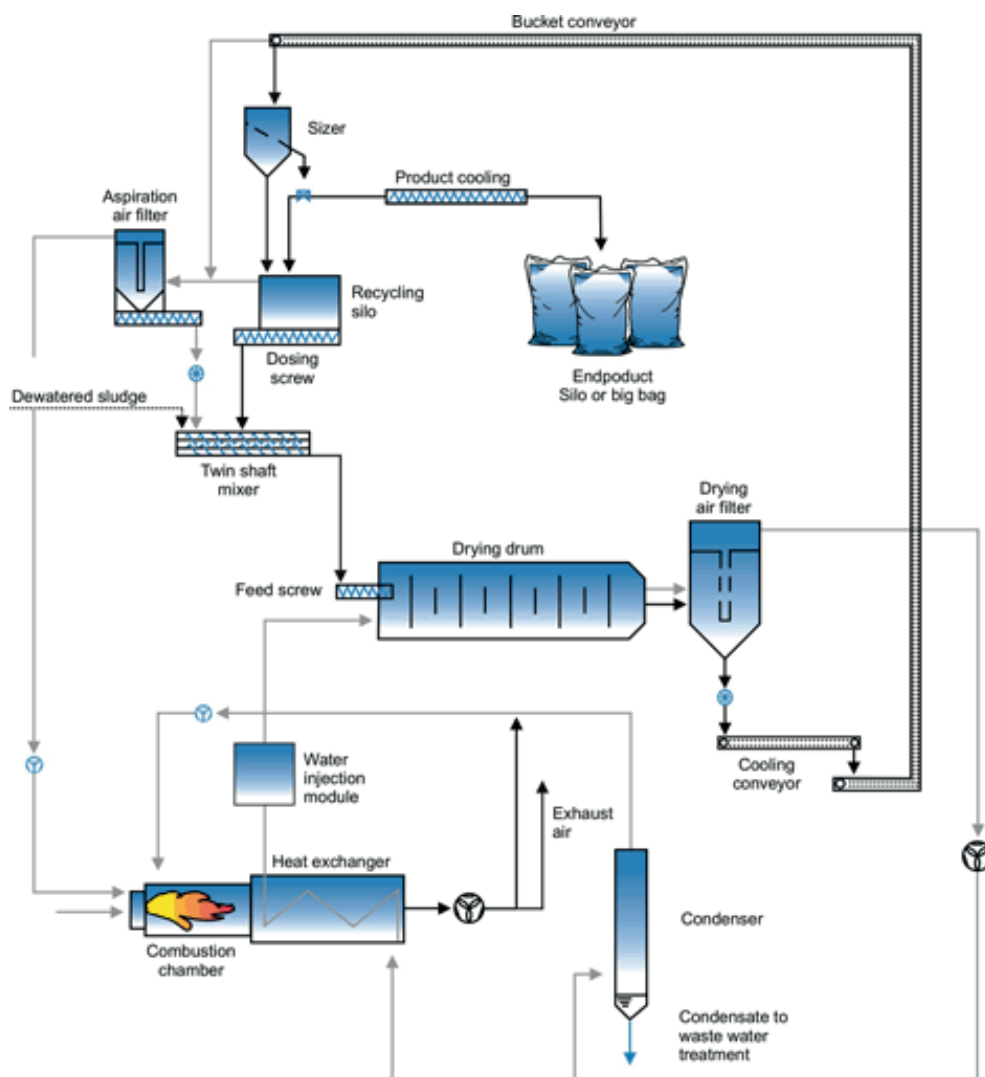
PROCES SC TECHNOLOGY SCHEMATISCH
