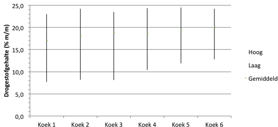
ONTWATERINGSRESULTAAT REFERENTIEMETING ZONDER GRUIS VAN VERSCHILLENDE KAMERS
