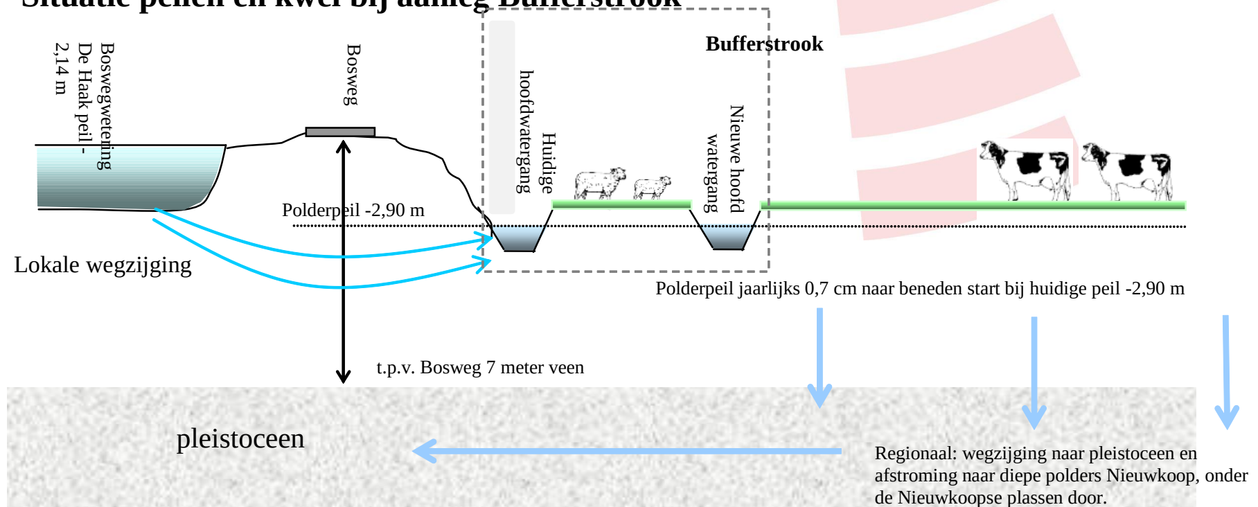
Afbeelding B2: Schematische weergave gewenste situatie met bufferzone
