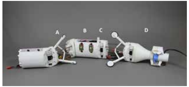
Figuur 3 Huidige prototype inspectierobot, met daarin klemmodules (A), modules voor elektronica (B), actuatoren voor beweging (C), propellermodule met camera en verlichting (D)
