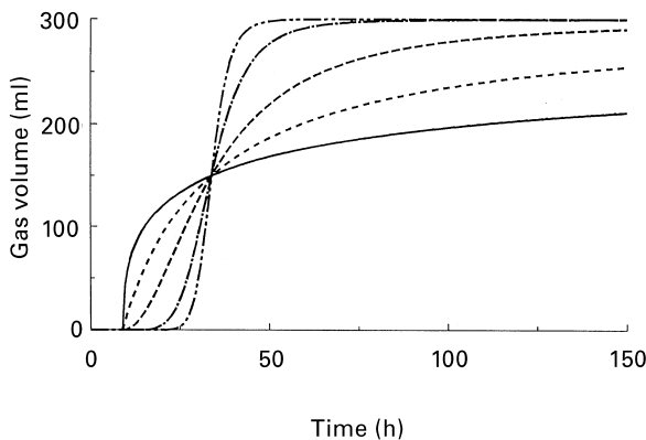
Fig. 4. The range of behaviour of the generalized Michaelis-Menten model with Y=500 ml/g, S_0=0.6 g, K=25 h and T=9 h. The parameter c is dimensionless. (—), c=0.5 ; (---), c=1 ; (---), c=2 ; (---), c=5 ; (---), c=10 .
