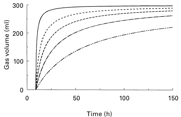
Fig. 5. The range of behaviour of the simple Michaelis-Menten model with Y=500 ml/g, S_0=0.6 g and T=9 h. The units of K are h. (—), K=1 ; (---), K=5 ; (---), K=10 ; (---), K=20 ; (---), K=50 .
