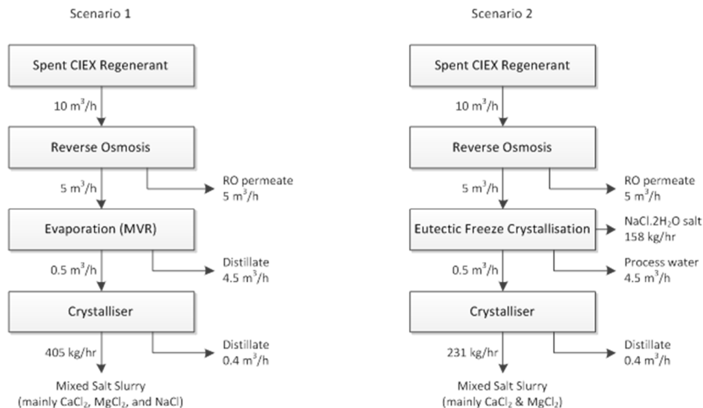
FIGUUR 1 SCENARIO'S VOOR ZUIVERING VAN REGENERAAT IONENWISSELING
