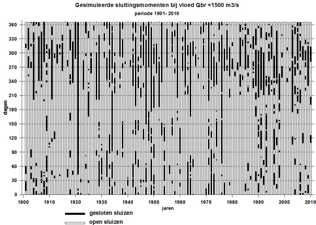
Figuur 3.2: Simulatie van de perioden van sluiting van de sluisen bij vloed op basis van de rivierafvoer bij Lobith van minder dan < 1500 m 3 /s (Paalvast, 2016).
