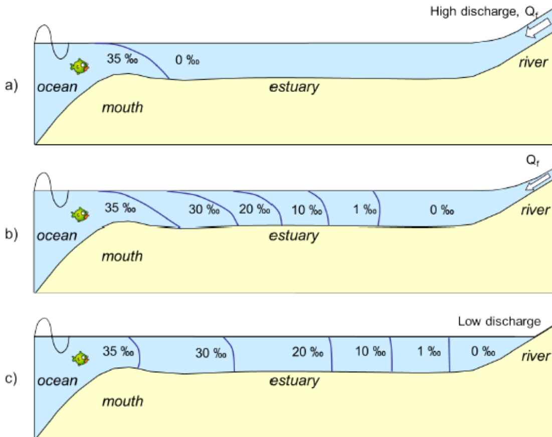
Figuur 3.4 Model weergave van de longitudinale verspreiding van het zoutgehalte (saliniteit) in een (a) gestratificeerd estuarium, (b) gedeeltelijk gemixt en (c) goed gemixt estuarium (Savenije 2012).
