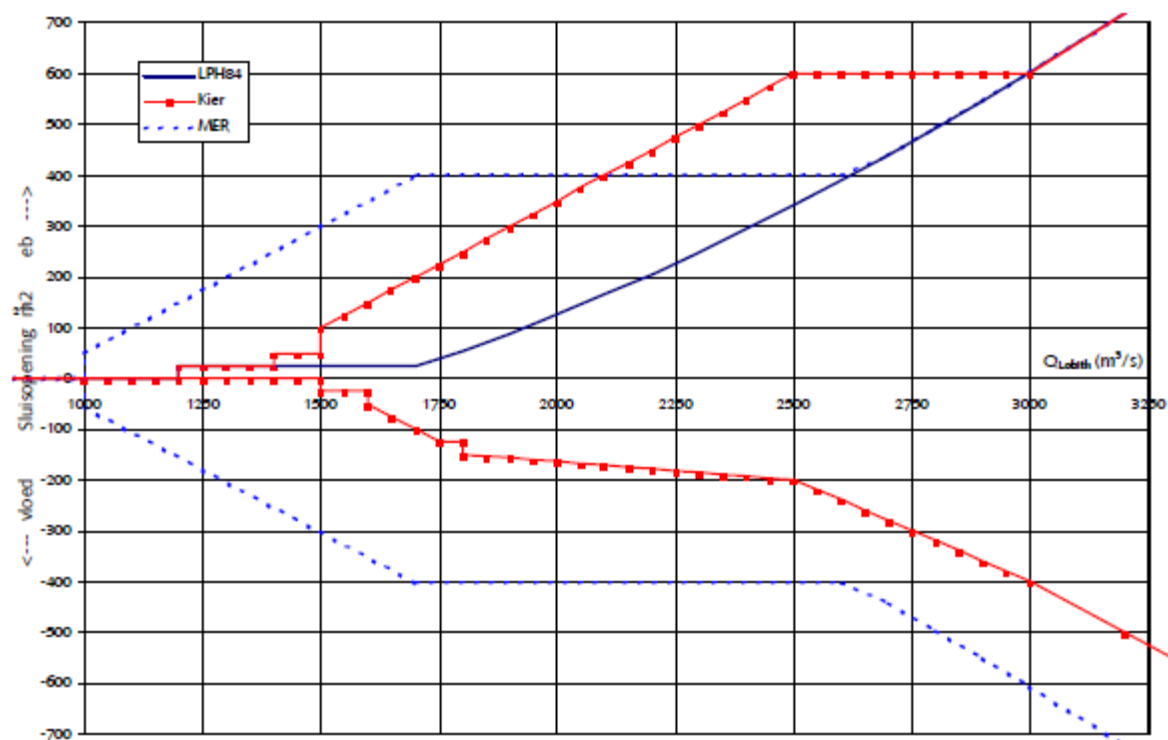
Figuur 3.2: De opening van de Haringvlietsluizen gerelateerd aan de Rijnafvoer bij Lobith. Kier beheersprogramma HOP (rood), en oorspronkelijke programma LPH84 (blauw) (Leeuwen et al. 2004).
