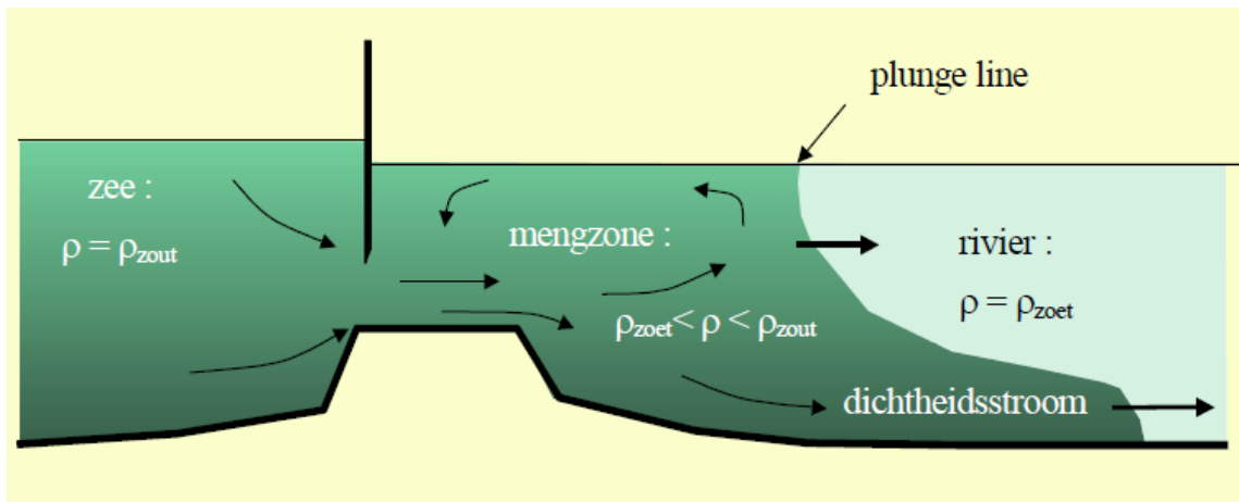
Figuur 3.5: Schematische weergave van de verwachte passage van zeewater door de Haringvlietsluizen (uit Jacobs et al 2003).
