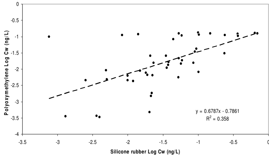
Figuur 4. Vergelijking van Cw voor PCBs, bepaald met POM-SPE en met siliconen rubber.
