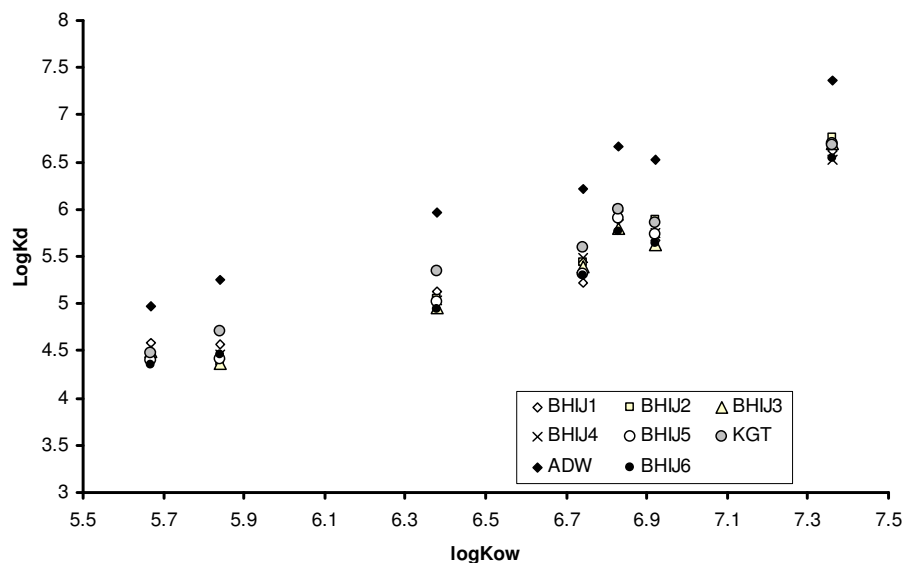
Figuur 6: Log Kd versus LogKow plots voor native PCBs. Cw bepaald met POM-SPE.
