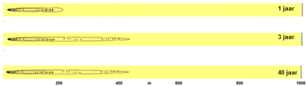
FIGUUR 5.5: GEMODELEERDE VERSPREIDING (49) VAN WARMTE IN DE RICHTING VAN GRONDWATERSTROMING (VAN LINKS NAAR RECHTS) MET EEN SNELHEID VAN 32CM/DAG (117M/JAAR) VOOR VERSCHILLENDE TIJDEN NA AANVANG WARMTEUITSTRALING DOOR EEN PUT VAN 80°C. DE BUITENSTE CONTOUR GEEFT 13°C WEER. AFSTANDEN ZIJN IN METERS VANAF DE PUT.
