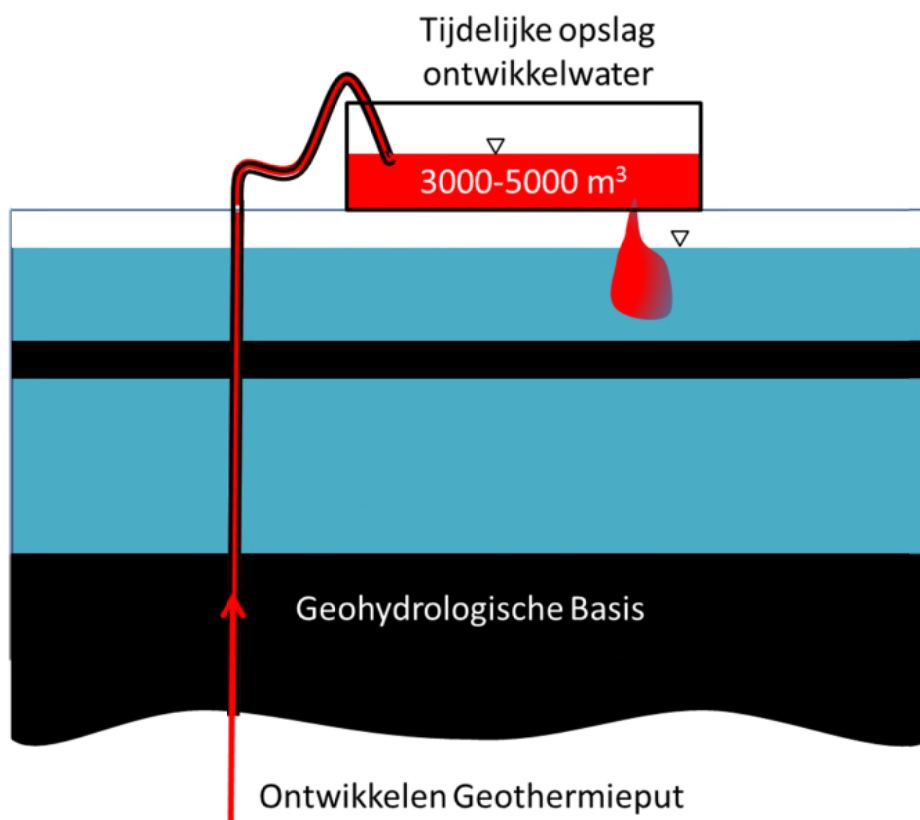
FIGUUR 4.6: SCHEMATISCHE WEERGAVE VAN TIJDELIJKE OPSLAG VAN WATER DAT VRIJKOMT TIJDENS HET ONTWIKKELEN VAN EEN GEOTHERMIEPUT. TER ILLUSTRATIE VAN HET RISICO VAN VERONTREINIGING VANAF MAAIVELD IS EEN LEKKAGE VANUIT DE OPSLAG ALS VOORBEELD WEERGEGEVEN.
