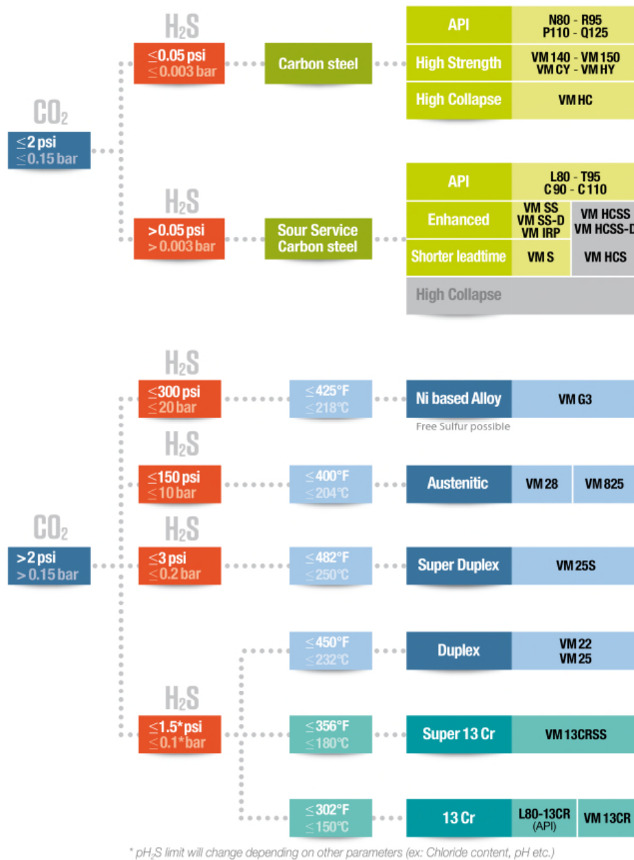
FIGUUR 4.10 VOORBEELD VAN EEN DIAGRAM VOOR STAALSELECTIE OP BASIS VAN CO 2 - EN H 2 S CONDITIES (BRON: WWW.VALLOUREC.COM ). KOOLSTOFSTAALSOORTEN WAARONDER L80 VALLEN IN DE GROEPEN BOVENAAN WEERGEGEVEN IN GROEN.
