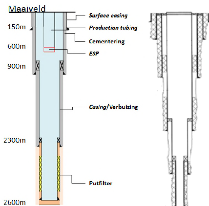
FIGUUR 4.8: LINKS: VOORBEELD VAN OPBOUW VAN EEN GROTENDEELS ENKELWANDIGE GEOTHERMIEPUT IN NEDERLAND (LINKS) MET GEBRUIKTE BENAMINGEN VOOR PUTONDERDELEN ( ESP : ELECTRICAL SUBMERSIBLE PUMP ). INDICATIEVE DIEPTEN BENEDEN MAAIVELD STAAN AANGEGEVEN. RECHTS: TER VERGELIJKING EEN VOORBEELD VAN DE TOT OP GROTE DIEPTE MEERWANDIGE CONSTRUCTIE VAN EEN GAS PUT IN NEDERLAND
