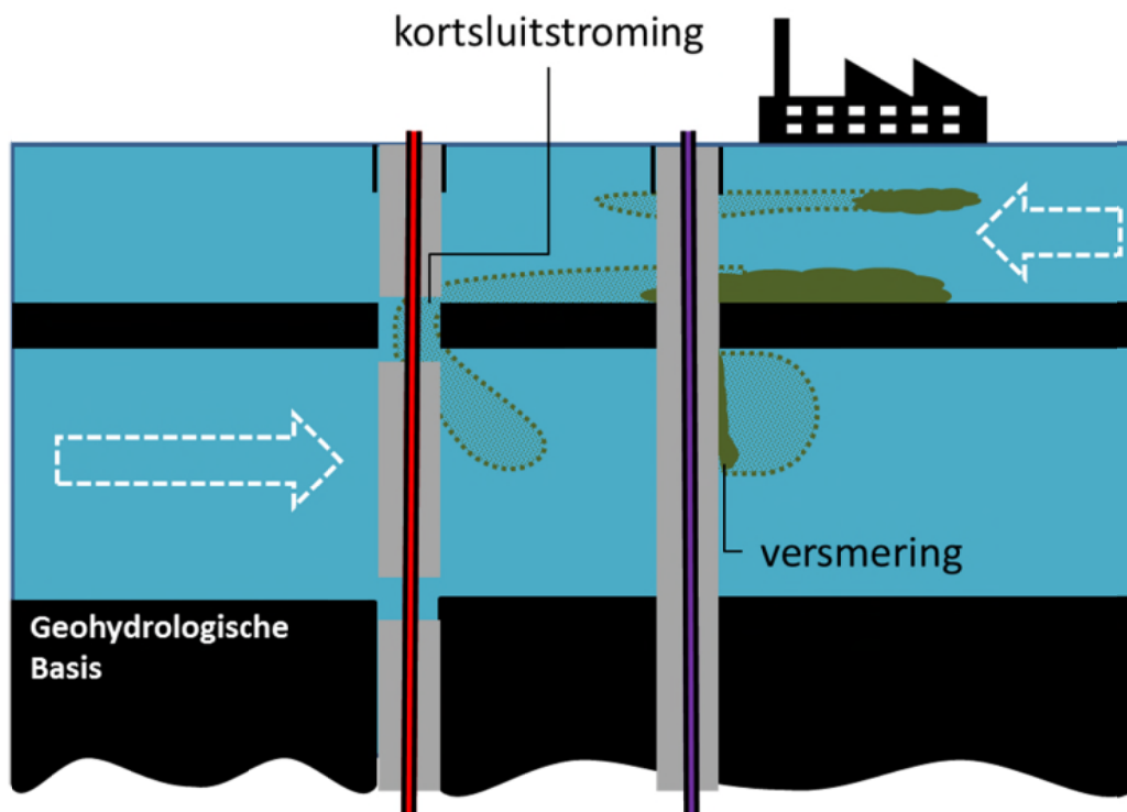
FIGUUR 2.4: SCHEMATISCHE WEERGAVE VAN VOORBEELDEN VAN RISICO'S OP VERONTREINIGING BIJ DOORBORING VAN GRONDWATERLAGEN DOOR KORTSLUITSTROMING ALS GEVOLG VAN ONVOLDENDE BOORGATAFDICHTING (GRIJS) VAN EEN SCHEIDENDE LAAG (LINKS) EN DOOR VERSMERING VAN BOVENLIGGENDE ZAKLAGEN (OLIJFGROEN). DE PIJLEN GEVEN ILLUSTRATIEF DE GRONDWATERSTROMING WEER.
