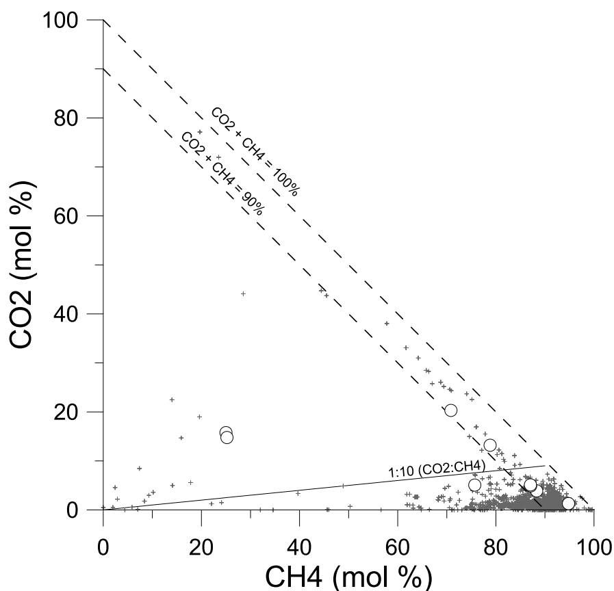
FIGUUR 4.4: DE MOLFRACTIES AAN CO 2 UITGEZET TEGEN METHAAN (CH 4 ) VAN GEOTHERMIESYSTEMEN IN NEDERLANDS (OPEN CIRKELS) UIT VERSCHILLENDE ONDERZOEKEN, WAARONDER (1). TER VERGELIJKING ZIJN DE GEMETEN FRACTIES IN GAS IN NEDERLANDSE OLIE- EN GASPUTTEN (GRIJZE PLUSJES, BRON:NLOG.NL) WEERGEGEVEN.
