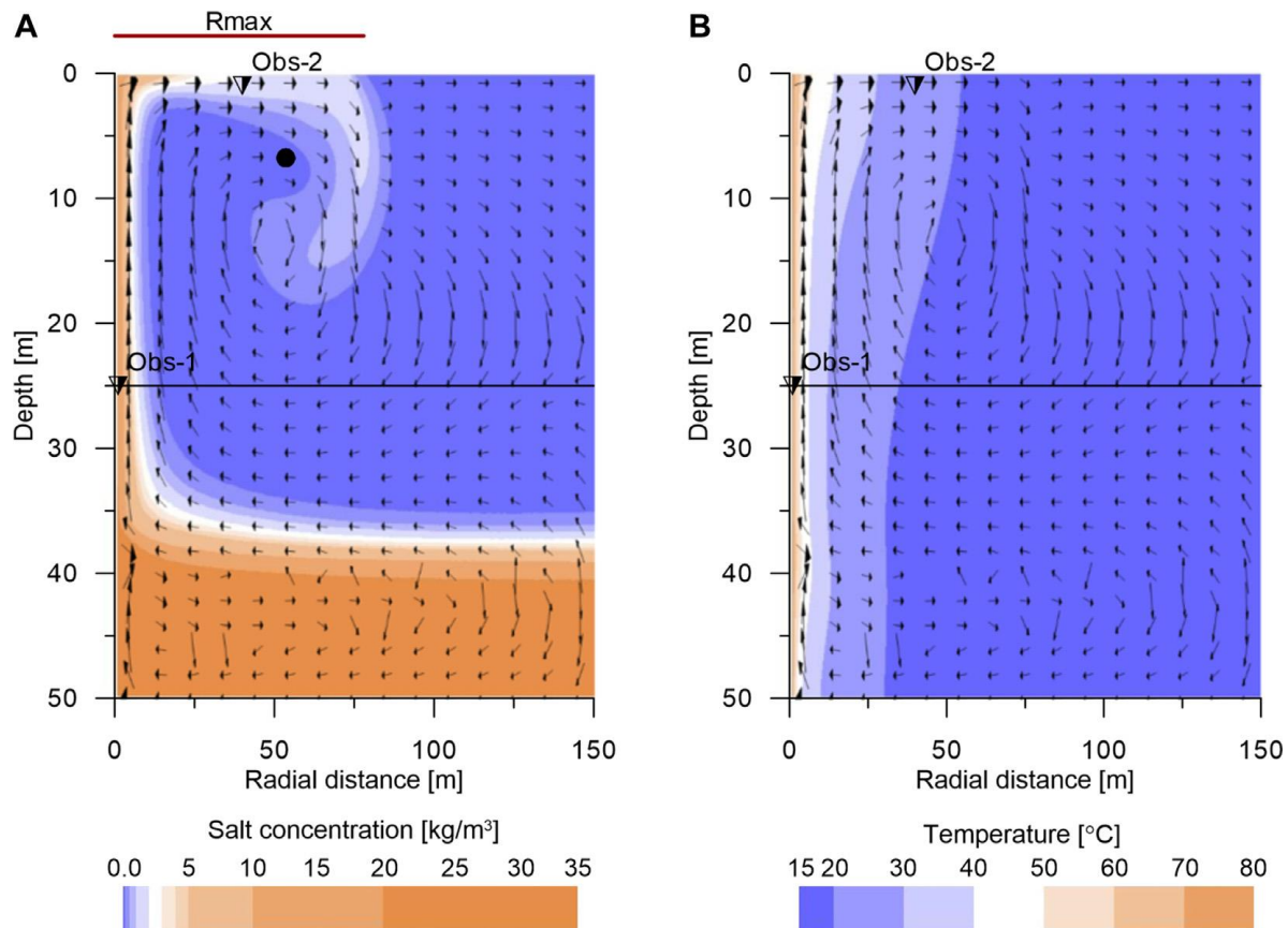
Afbeelding 3. Zoutconcentratie (A) en temperatuur (B) rondom een geothermieput ter plaatse van een doorboorde aquifer [13]
