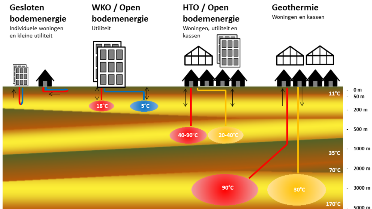
Afbeelding 1. Schematisch overzicht van typen bodemenergiesystemen met meest voorkomende toepassingsgebieden en natuurlijke en brontemperaturen
