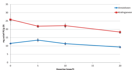
AFBEELDING 10 BENODIGDE PE-DOSERING BIJ SLIB VAN RWZI KRALINGSEVEER EN RWZI AMSTELVEEN BIJ VERSCHILLENDE DOSERINGEN VAN \text{Fe}^{3+}
