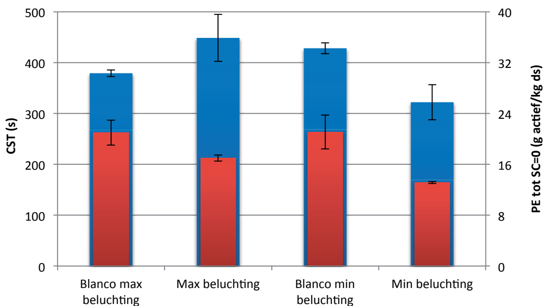
AFBEELDING 27 RESULTATEN ONTWERINGSPROEVEN OP LABSCHAAL VOOR MONSTERS VAN DE RWZI AMSTERDAM W. LINKERAS: CST RESULTATEN, RECHTERAS: PE TITRATIE TOTDAT DE STREAMING VOLTAGE NUL IS
