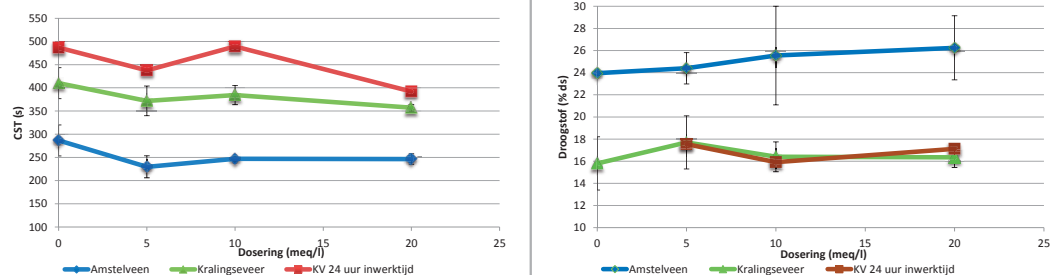
AFBEELDING 4A CST EN 4B DS% VAN UITGEGIST SLIB VAN RWZI KRALINGSEVEER EN RWZI AMSTELVEEN BIJ VERSCHILLENDE DOSERINGEN VAN Mg^{2+}
