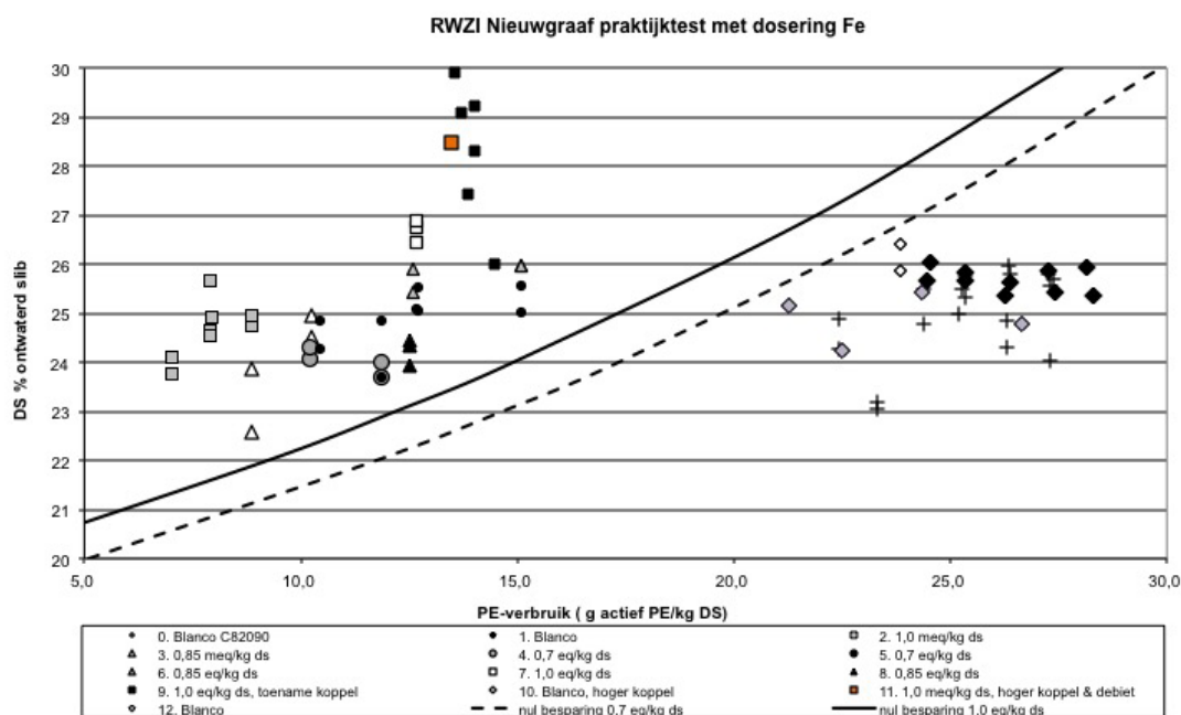
AFBEELDING 22 ONTWATERINGSRESULTATEN PRAKTIJKPROEF NIEUWGRAAF. DE VERSCHILLENDE SYMBOLEN GEVEN VERSCHILLENDE DAGEN EN CONDITIES WEER. ALLEEN PROEF 0 IS MET PE C82090 UITGEVOERD (SYMBOL: +). ALLE ANDERE RESULTATEN ZIJN MET PE SD 2081
