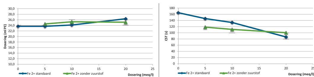
AFBEELDING 7A CST EN 7B DS% VAN SLIB VAN RWZI KRALINGSEVEER EN RWZI AMSTELVEEN BIJ VERSCHILLENDE DOSERINGEN VAN \text{Fe}^{2+} ONDER ZUURSTOFLOZE EN STANDAARDOMSTANDIGHEDEN (MET ZUURSTOF)
