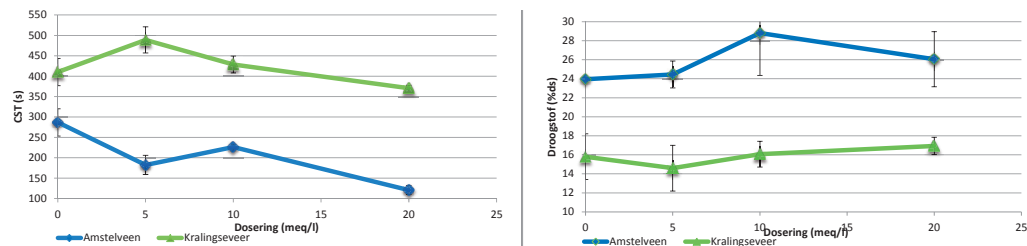
AFBEELDING 6A CST EN 6B DS% VAN SLIB VAN RWZI KRALINGSEVEER EN RWZI AMSTELVEEN BIJ VERSCHILLENDE DOSERINGEN VAN \text{Fe}^{2+}
