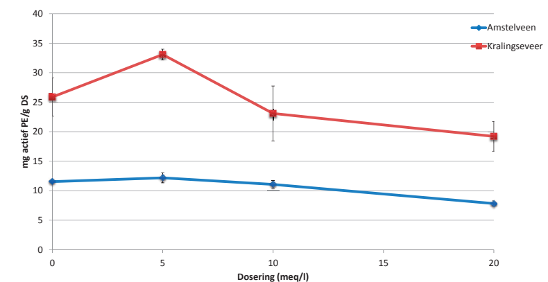
AFBEELDING 8 BENODIGDE PE-DOSERING BIJ SLIB VAN RWZI KRALINGSEVEER EN RWZI AMSTELVEEN BIJ VERSCHILLENDE DOSERINGEN VAN \text{Fe}^{2+}
