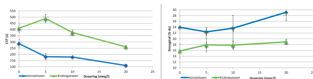
AFBEELDING 9A CST EN 9B 5% VAN SLIB VAN RWZI KRALINGSEVEER EN RWZI AMSTELVEEN BIJ VERSCHILLENDE DOSERINGEN VAN \text{Fe}^{3+}
