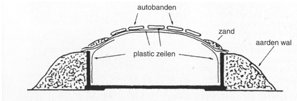
Figuur 11.4 Wijze van afdekken van een sleufsilos met uitsluitend plastic
