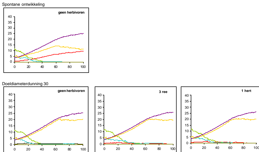
Figuur 4.9: Verloop van de verdeling van grondvlakken (m 2 per ha) in het bostype Gemengd bos op holtpodzol over een periode van 100 jaar bij het beheersscenario doeldiameterdunning 30 t.o.v. het beheer van nietsdoen. De dichtheden van de herbivoren zijn aangegeven in de sub-figuren. De legenda van de boomsoorten kunt u vinden op de laatste pagina van het rapport.
