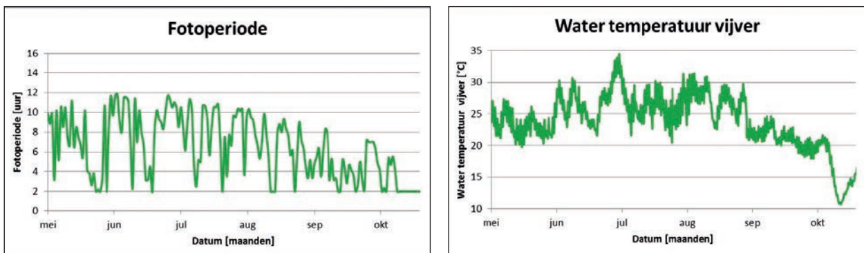
Figuur 3: Gemeten fotoperiode en watertemperatuur van de kroosvijver voor de maanden mei tot en met oktober 2015. De optima voor de fotoperiode en watertemperatuur zijn respectievelijk 13 [uur] en 26 [°C].
