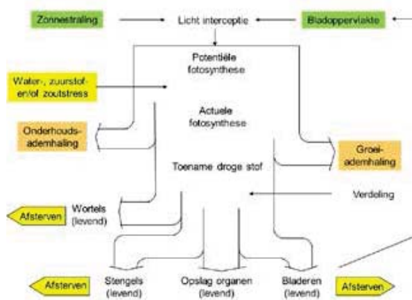
Stroomschema van gewasgroeiprocessen in WOFOST
