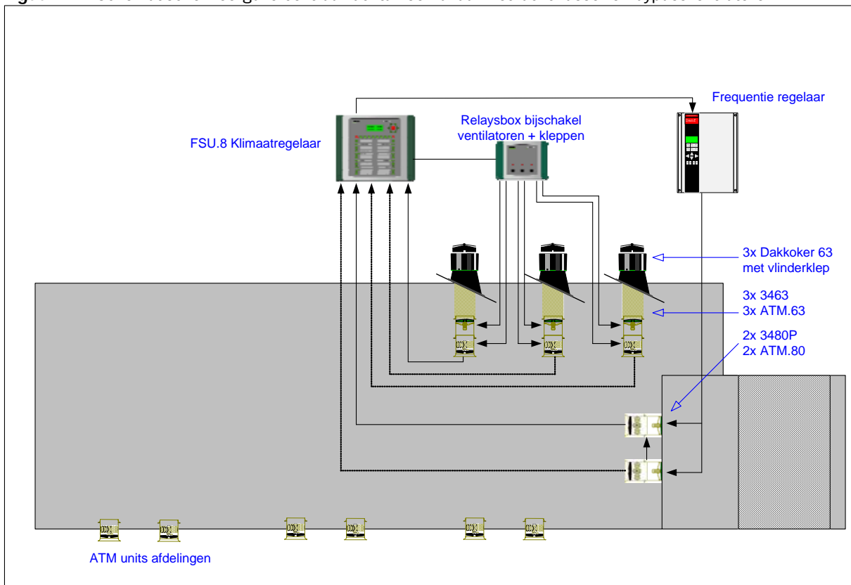
Figuur 2 Schematische weergave centraal luchtafvoerkanaal met luchtwasser en bypassventilatoren
