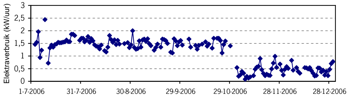
Figuur 5 Gemiddeld elektraverbruik per dag (kW/uur) van de ventilatoren bij de luchtwasser
