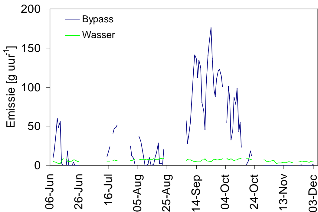
Figuur 4 NH 3 -emissie door de bypassventilatoren en door de wasser (semicontinu metingen)
