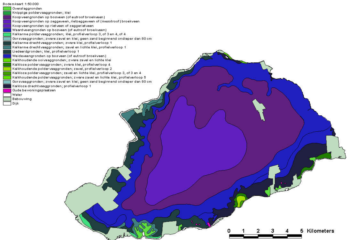
Figuur 4. Bodemkaart 1:50.000 van de Krimpenerwaard (Steur & Heijink, 1991)
