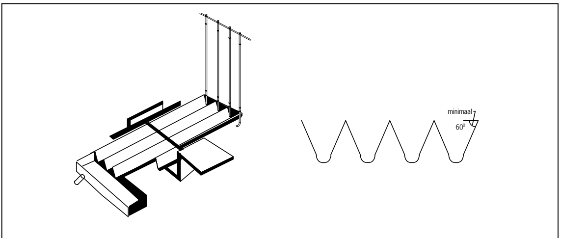
Figuur 2 Spoelgotensysteem
