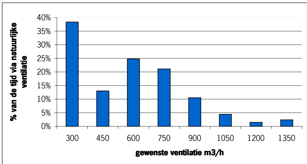
Figuur 4 Percentage van de tijd dat gemiddeld over ronde 3 t/m 7 volledige natuurlijke ventilatie werd geregistreerd bij de verschillende ingestelde gewenste ventilatiehoeveelheden per uur
