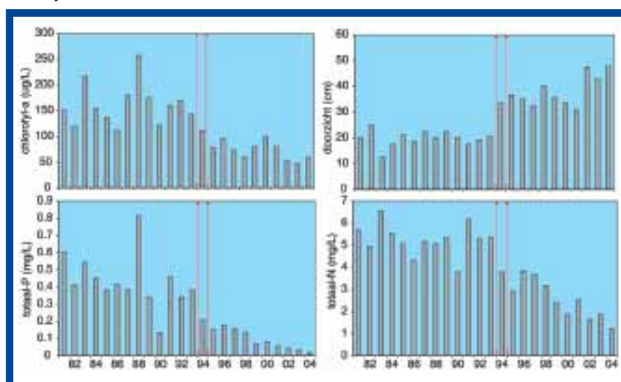
Afb. 2: Verloop van zomergemiddelden van totaal fosfaat, doorzicht chlorofyl-a en totaal stikstof in het Nannevijf
