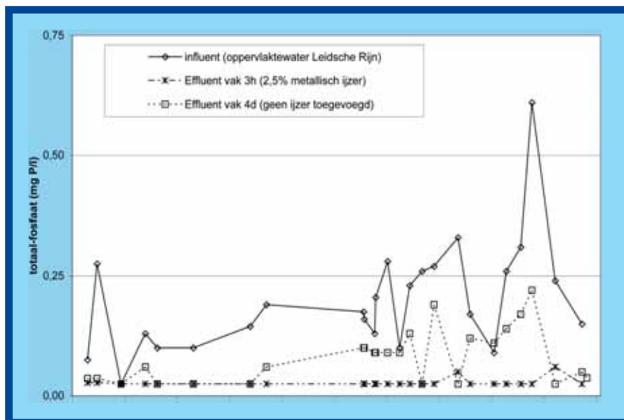
Afb. 1: Het verloop van het fosfaatgehalte in het influent en effluent in twee proefvakken.
