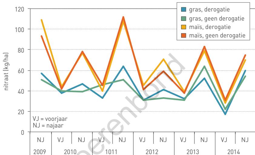
Figuur 1 Gemiddeld nitraatstikstofgehalte in de bodemlaag 0-90 cm (kg NO 3 -N/ha) op gras- en maïspcelen in het derogatieproject op zandbodems, op verschillende tijdstippen in de periode 2009-2014 - Bron: BDB
