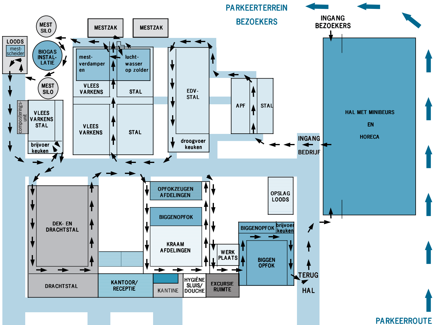
Economisch duurzame vleesvarkensstal
