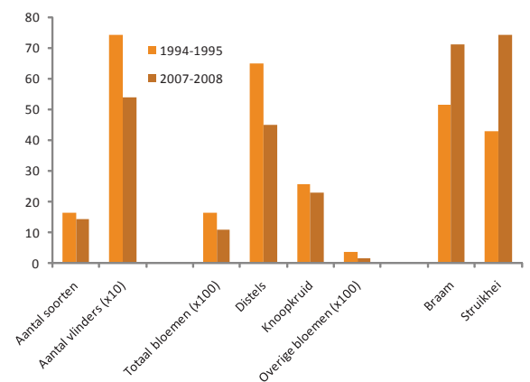
Figuur 2: Veranderingen in de vlinderstand (aantal soorten per route en aantal vlinders per sectie van 50 m) en het bloemenaanbod langs Nederlandse vlinderroutes tussen 1994-1995 en 2007-2008 (bloemenaanbod in aantal bloemen, bloemhoofdjes of -aren per sectie van 50 m, gemiddelde over een heel seizoen); alle verschillen zijn statistisch significant ( P < 0,05 ).
