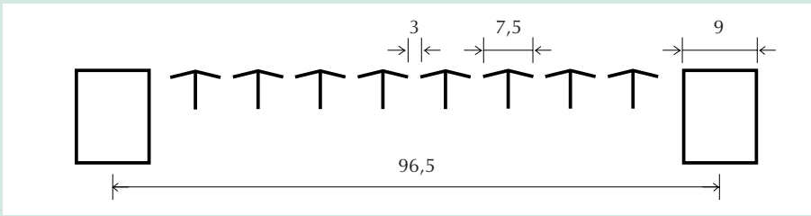
Figuur 4 Vorm en afmetingen (cm) van de stalen roosters
