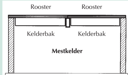
Figuur 5 Schematische doorsnede mestgang met stalen roostervloersysteem
