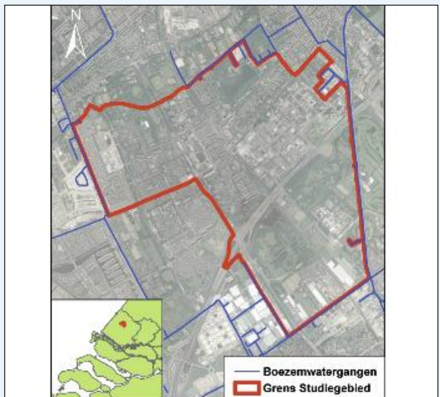
Afb. 1: Het studiegebied de Plaspoel- en Schaapweipolder met een oppervlakte van 751 hectare. De aangrenzende boezemkade is 81 km lang.
