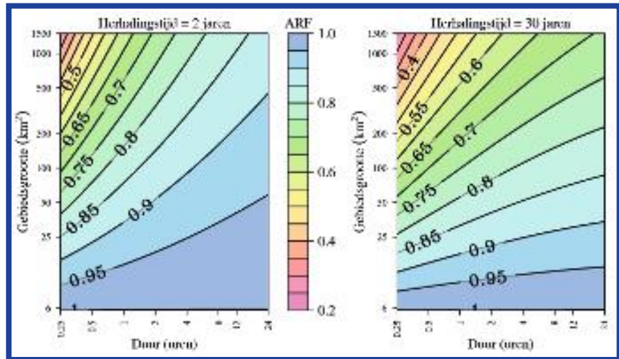
Afb. 1: Gebiedsreductiefactor (areal reduction factor of ARF) voor een herhalingsstijd van twee jaar (links) en 30 jaar (rechts).
