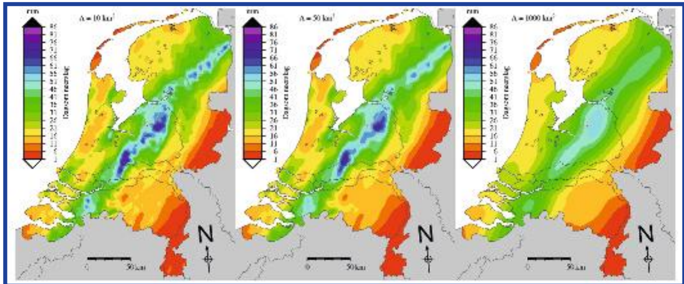
Afb. 2: Neerslag van 12 juli 2011, 10.00 uur tot en met 13 juli 2011, 10.00 uur voor gebieden van tien km 2 (links), 50 km 2 (midden) en 1.000 km 2 (rechts). Gebaseerd op radar data.
