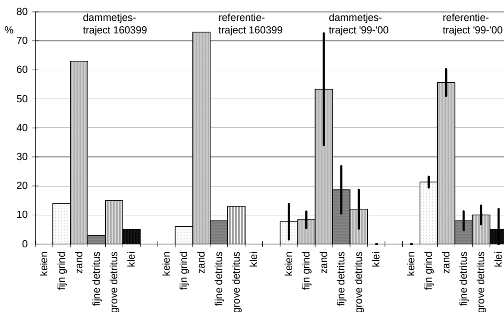
Figuur 38. De procentuele verhouding van de opbouw van het bodemprofiel in het dammetjes- en referentietraject voor en na aanleg van de keiendammetjes
