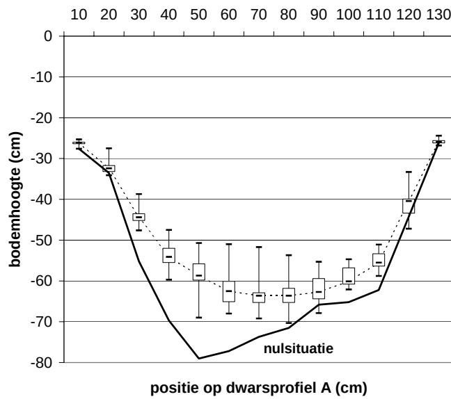
Figuur 17. Boxplot van de beekbodemhoogte (negatieve afstand ten opzichte van de meetbuis) op permanent dwarsprofiel A over de gehele meetperiode. De nulsituatie is gebaseerd op de steekmonsters van 20 januari 2000
