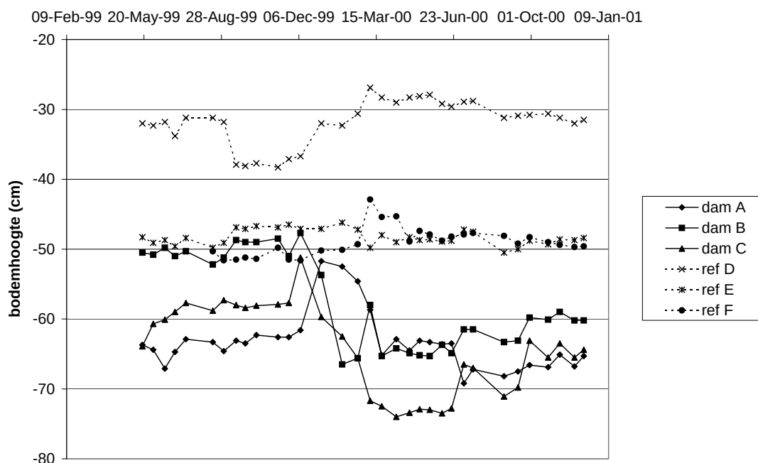
Figuur 23. De beekbodemhoogte (negatieve afstand ten opzichte van de meetbuis) gemeten in het midden van ieder permanent dwarsprofiel
