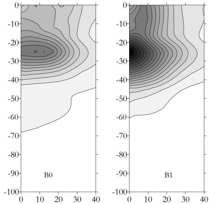
Figuur 11 Verdeling van de cumulatieve opname over het bodemprofiel bij wel (B1) en niet (B0) beregenen bij volheids dieper ondergewerkt (P2) en een smal en diep wortelstelsel (W1) Hoe donkerder, des te groter de opname.
