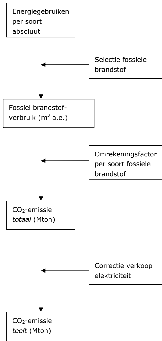
Figuur 2.2 Schematische weergave bepaling CO 2 -emissie glastuinbouw.
