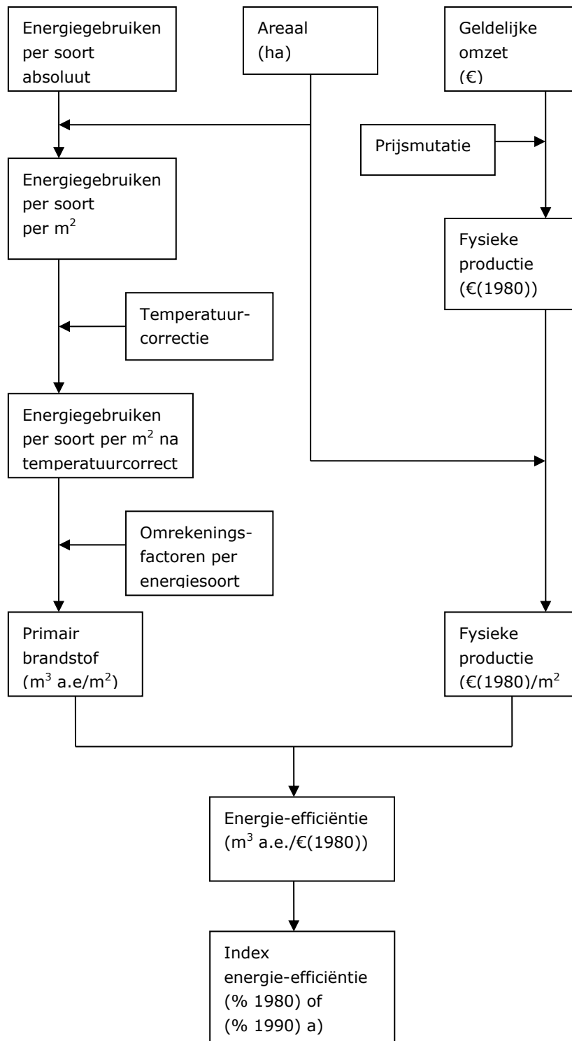
Figuur 2.1 Schematische weergave bepaling energie-efficiëntie productieglastuinbouw. a) Afhankelijk van het basisjaar waarin de energie-efficiëntie wordt uitgedrukt; vanaf 2009 is dit (% 1990).
