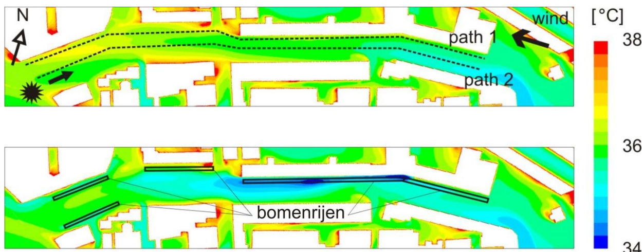
Figuur 3.7 Luchttemperatuur op voetgangershoogte (2 m boven de grond) in de J.P. van Muijlwijkstraat in Arnhem voor de huidige situatie (boven) en voor het scenario met bomenrijen in de gehele straat (onder). De bomenrijen zijn weergegeven door de zwarte rechthoeken (Gromke et al., 2015).
