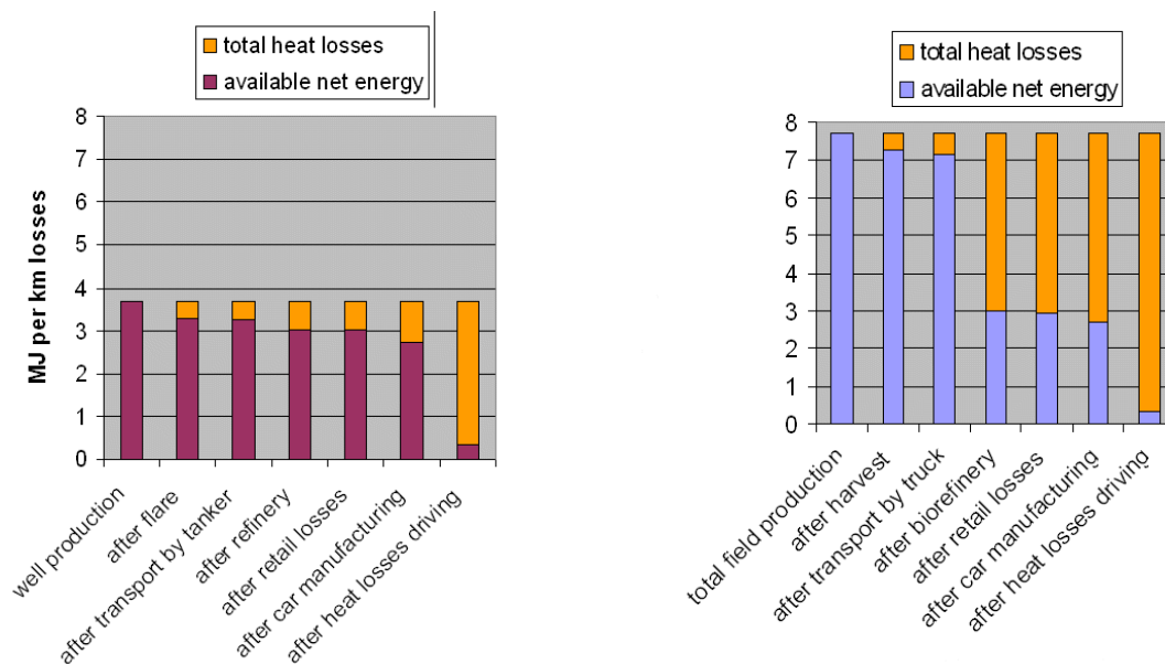
Figuur 10: Cascades (vervalstappen) in de 'Well-to-Wheel'-keten (links) en de 'Crop-to-Craft'-keten (rechts).
