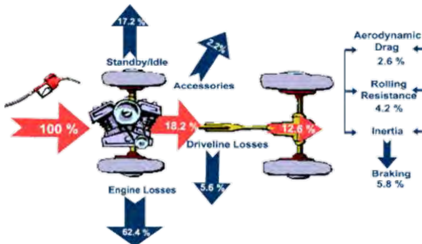
Figuur 9: Energiestromen in een automobiel met zuigermotor.
