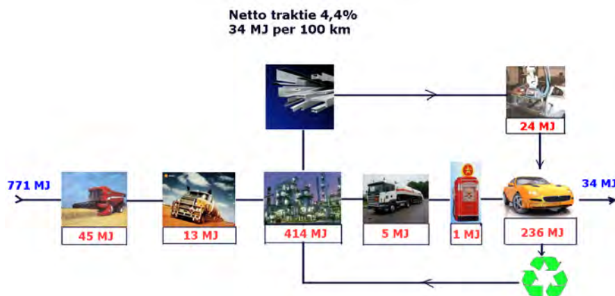
Figuur 3: Crop-to-Craft-analyse voor automobieltransport. Voor 100 km voortstuwing is 34 MJ voortstuwingsenergie nodig, waarvoor in de fossiele keten 428 MJ olie uit een bron moet worden gehaald (8% rendement). In de biomassaketten moet 771 MJ biomassa aangemaakt worden voor eenzelfde prestatie (4% rendement).
