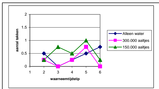
Figuur 3 Verloop van het aantal nieuw aangetaste takken per veld (ten opzichte van de voorgaande waarneming), zoals waargenomen.
