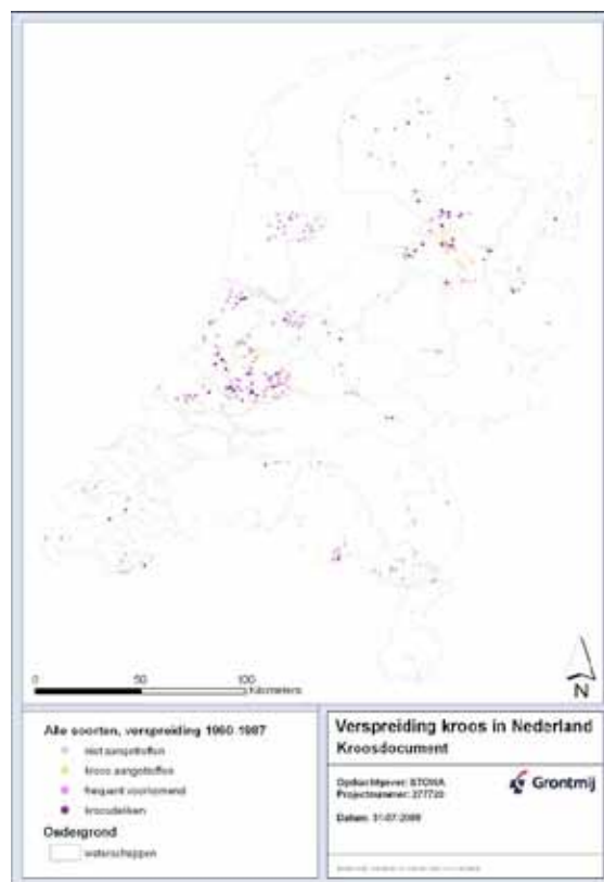
FIGUUR B1-1: ALLE SOORTEN 1960 T/M 1987
