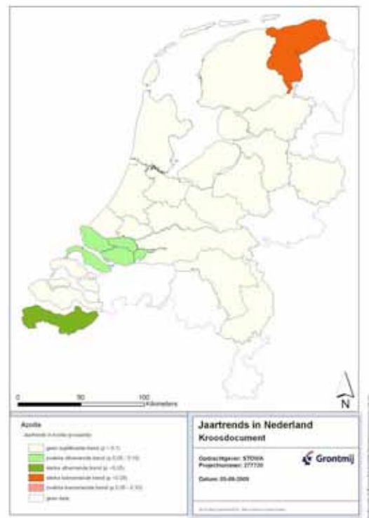
FIGUUR B2-2: JAARTRENDS VAN BEDEKKING AZOLLA FILICULOIDES (PERIODE 1980-2008)
