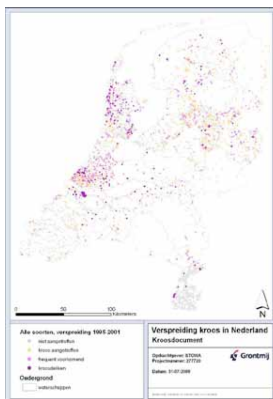
FIGUUR B1-3: ALLE SOORTEN 1995 T/M 2001
