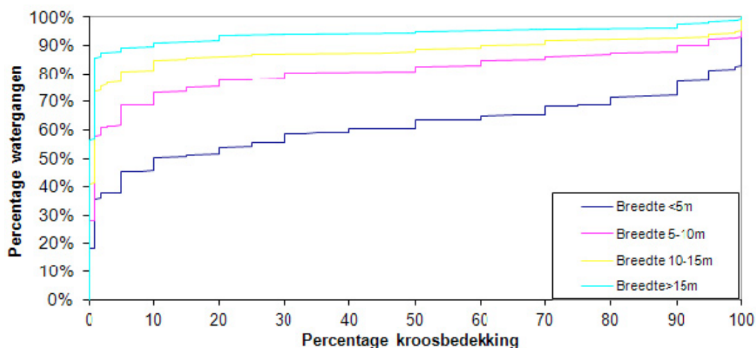
DE CUMULATIEVE FREQUENTIEVERDELING VAN DE BEDEKKING VAN KROOS IN RELATIE TOT DE BREEDTE VAN DE WATERGANG
