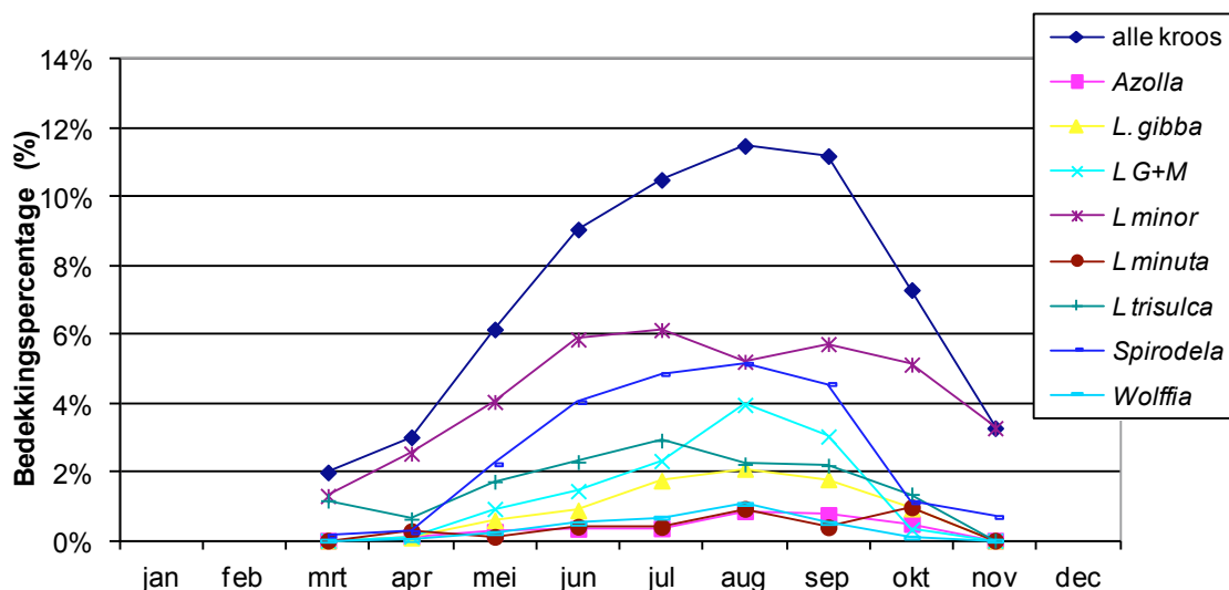
FIGUUR 3.3 GEMIDDELDE BEDEKKING VAN KROOS PER MAAND (PERIODE 1980-2008)
