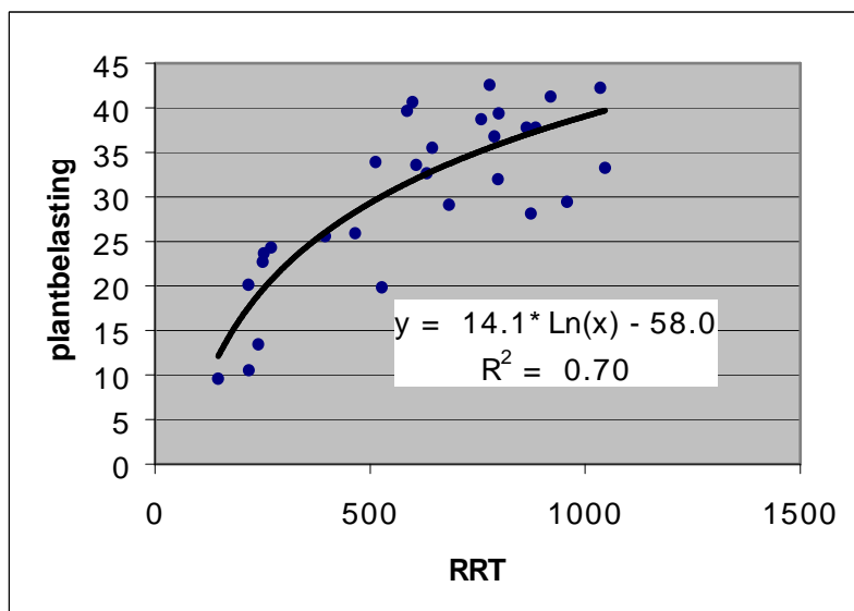
Figuur 4.4 - Verband tussen RRT ( J\text{ cm}^2\text{ }^\circ\text{C}^{-1} ) en plantbelasting (vruchten per \text{m}^2 in afdeling 4 voor het complete teeltseizoen. Voor overige details zie figuur 4.3.
