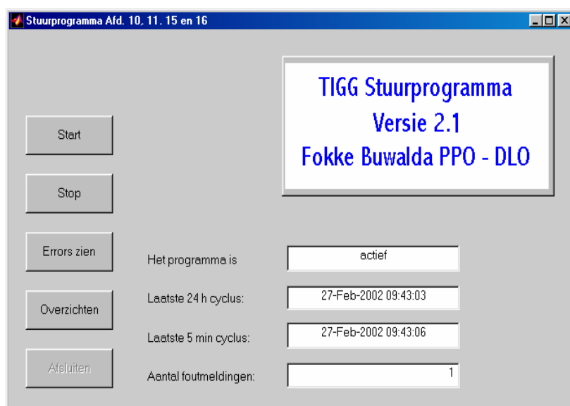
Figuur 5.2 - De interactieve gebruikersinterface van het stuurmodel waarmee de kasttemperatuur in vier afdelingen met paprika werd aangestuurd. Het model communiceerde met een Priva Integro en een Hoogendoorn Economic, waarop het klimaatprogramma Econaut CTI draaide. Foutmeldingen werden geregistreerd en konden worden bekeken door op de knop 'Errors zien' te klikken; de knop 'overzichten' opende een scherm met actuele waarden voor kasttemperatuur, setpoints, temperatuursommen, etc.
