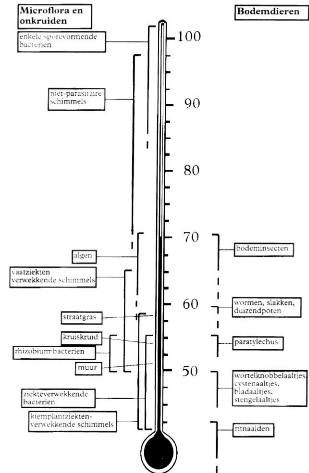
Dodingstemperaturen van microflora, onkruiden en bodemdieren bij een behandeling van de grond gedurende 30 minuten.
