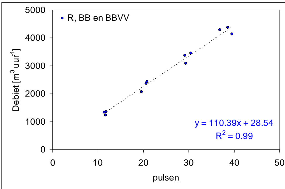
Figuur C2 Kalibratielijnen meetventilatoren op locatie 2. R: referentieafdeling; BB: afdeling met balansballen; BBVV: afdeling met balansballen en VevoVitall®
