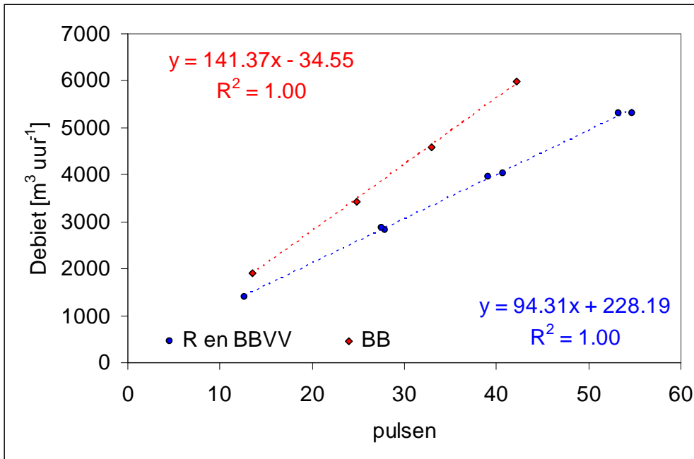
Figuur C1 Kalibratielijnen meetventilatoren op locatie 1. R: referentieafdeling; BB: afdeling met balansballen; BBVV: afdeling met balansballen en VevoVitall®
