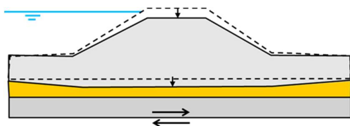
Figuur 4.8 Kruindaling door een combinatie van vervorming van de zandlaag (wegdrukken en compactie) en niet-doorgaande afschuiving.
