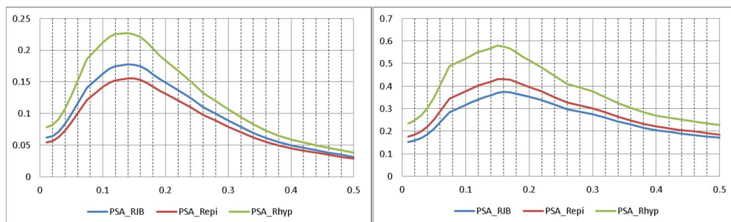
Figuur 1.9 Response spectra voor M = 3.5 en M = 5 aardbevingen, afschuiving zoals in Groningen (normal faulting), vlg. [Akkar et al 2013]
