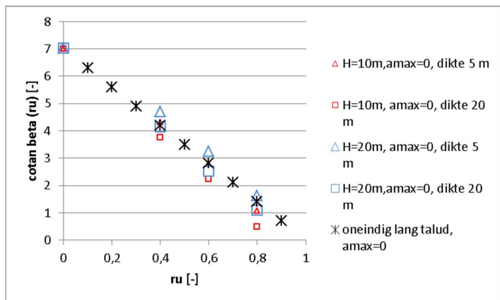
Figuur 0.11 Relatie equivalente taludversteiling en relatieve wateroverspanning (ru) in een 5 m en 20 m dikke laag voor een recht, onder water 1:7 zandtalud van 10 en 20 m hoog met sterkte \phi = 30^\circ , met een Bishop glijvlak. Tevens weergegeven zijn de resultaten van een oneindig lang 1:7 talud
