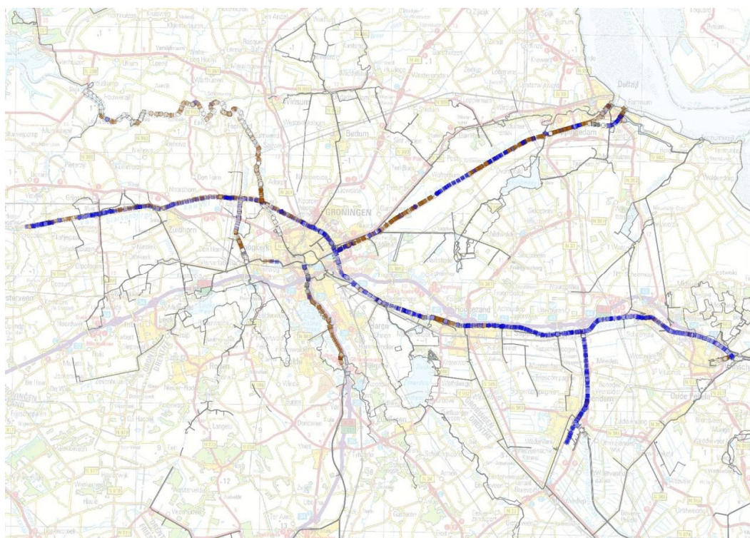
Figuur F.2 Bekende locaties voor beschoeiing (blauw is stalen damwand, bruin is houten beschoeiing, grijs is betonnen damwand, wit is overige) – Een beschoeiing tot in de deklaag is ook een criterium voor hydraulische kortsluiting
