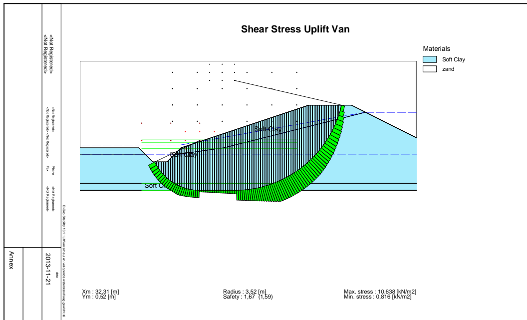
Figuur E.9 Glijvlak volgens Lift-Van, evenwichtsfactor = 1,59
