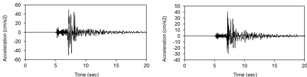
Figuur 2.6: Event 6: Huizinge, opnemer WSE, radiale component (links) en transversale component (rechts)
