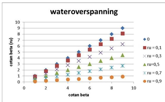
Figuur 0.4 Reductie van hellingshoek (cotan \beta ) ten gevolge van wateroverspanningen, gegeven een oneindig lang talud.
