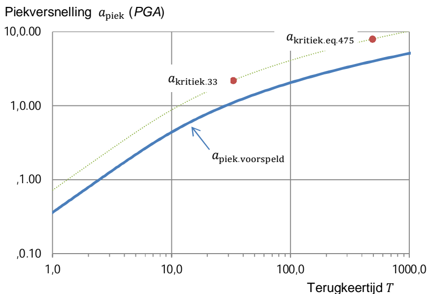
Figuur G.6: Voorbeeld van de bepaling van de equivalente kritieke piekversnelling bij een terugkeertijd van 475 jaar uit een berekende kritieke versnelling bij een terugkeertijd van 33 jaar
