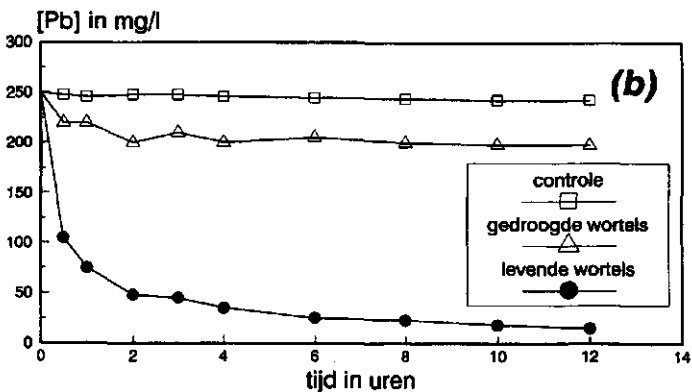
Figuur 4: Opname van Pb door Brassica juncea in een watercultuur (naar: Dushenkow et al., 1995). a: de relatie tussen de oorspronkelijke Pb-concentratie en de tijd die Brassica juncea nodig heeft om de Pb-concentratie in oplossing te halveren; b: een vergelijking tussen de effectiviteit van dood plantenmateriaal en levende planten.
