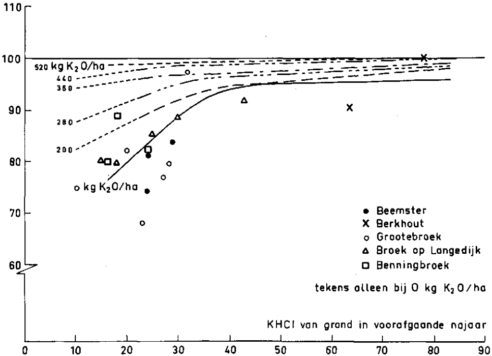
Fig. 1 Relatieve opbrengst van vroege aardappelen in afhankelijkheid van K-HCl van de grond.
