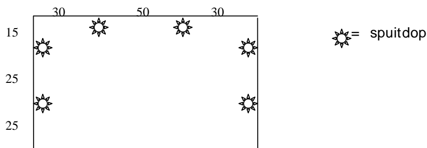
Figuur 6. Opzet van de spuitwagen.
