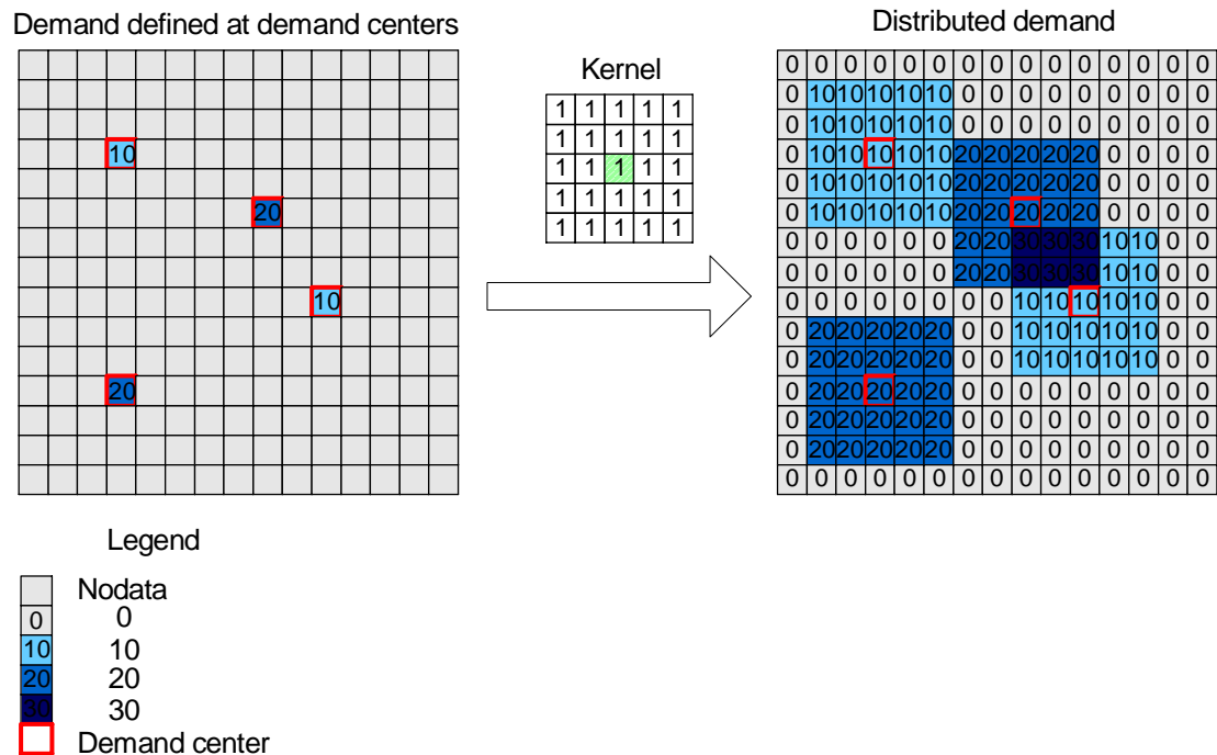
Figure 4.4. Verdelen van de vraag m.b.v. Kernel Convolutions
