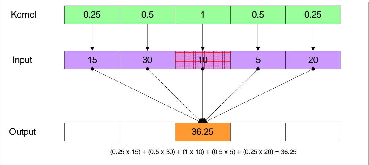
Figuur 4.3 Rekenvoorbeeld Kernel Convolution (gewichten als functie van de afstand tot de middelste cel)
