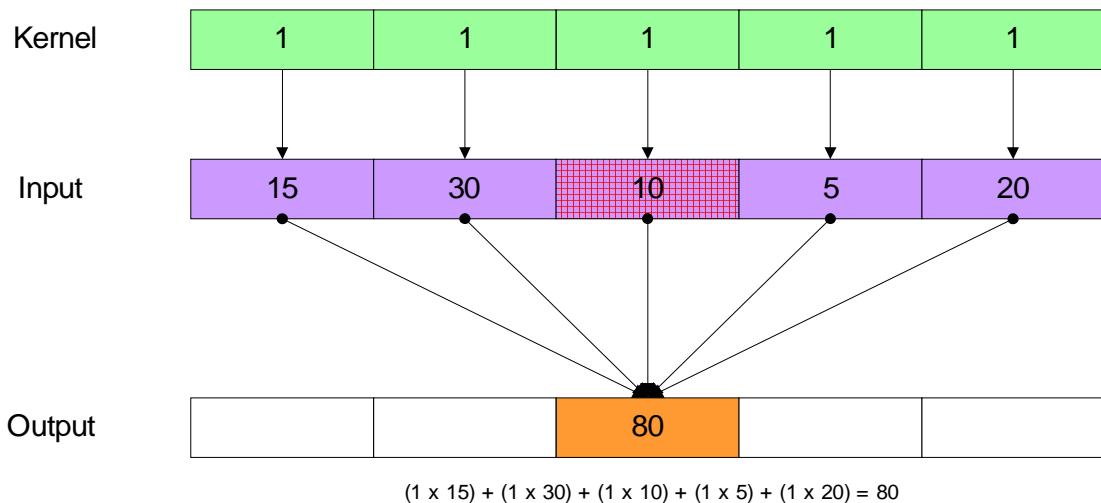
Figuur 4.2. Rekenvoorbeeld Kernel Convolution (uitgevoerd als Focal Sum)
